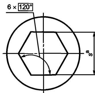
Рисунок С.1 — Калибр для проверки допуска формы, установленного на рисунках 23, 71 и 94.
