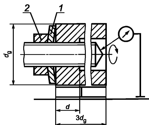
1 — коническая пружинная шайба калибра; 2 — контргайка калибра
