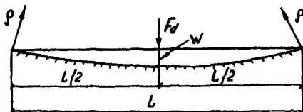
Рис. 1. Схема расчета кривизны изгиба плиты
