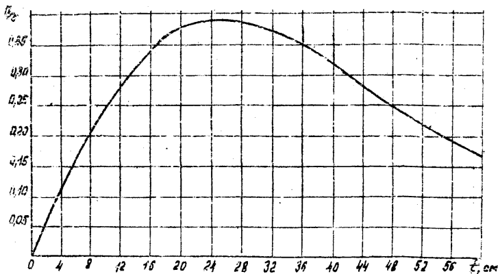
Рис. 6. Изменение параметра \alpha_3 в зависимости от толщины покрытия
