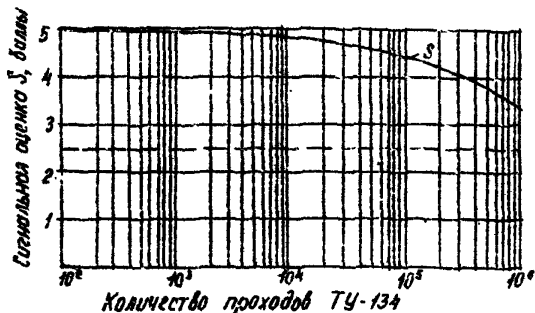
Рис. 2. Определение предельно допустимого количества проходов самолета Ту-134 в зависимости от сигнальной оценки \bar{S} .
