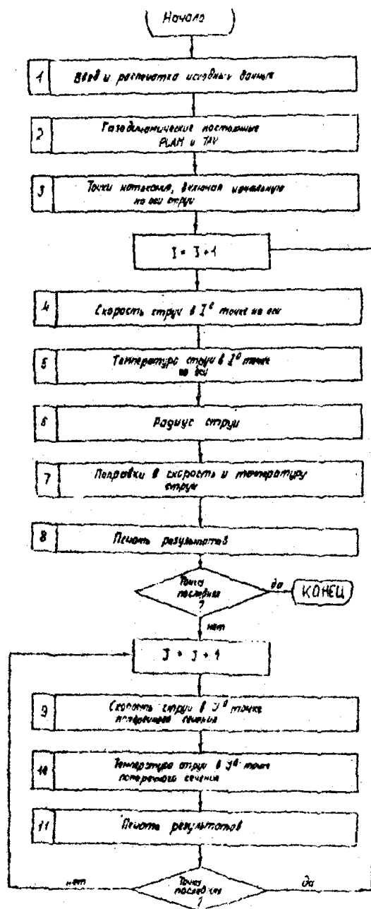
Рис. 7. Блок-схема расчета температур и скоростей в поле струи расчетного двигателя
