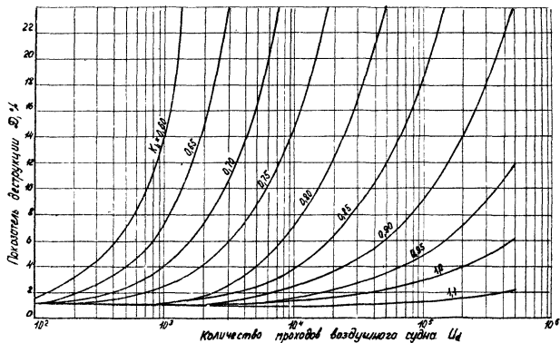
Рис. 4. Кривые деструкции D = 1 + \exp(3.1 - 15.4 K_u) (\lg U_d)^3 для различных коэффициентов K_u
