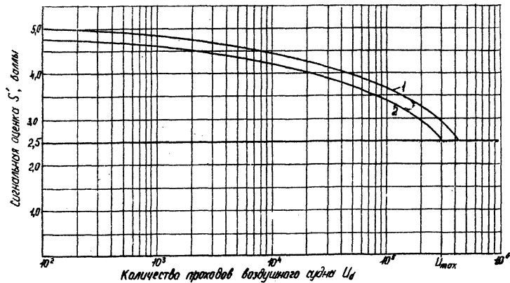
Рис. 5. Определение предельно допустимого количества проходов воздушного судна U_{\text{max}} : 1, 2 - кривая сигнальной оценки покрытия соответственно для сквозных трещин и с учетом сколов кромок.
