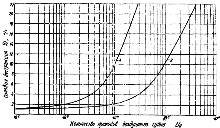
Рис. 3. Зависимость силовой деструкции для ряда плит (1) и для змей ВПШ (2) от количества проходов расчетного типа воздушного судна
