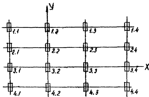
Рис. 9. Схема координат многоколесных шасси
