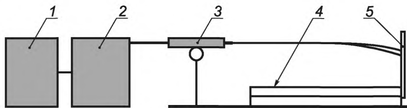
1 — емкость с пенообразователем; 2 — насосная установка; 3 — пенный ствол; 4 — противень с горячей жидкостью; 5 — экран для сбора пены
