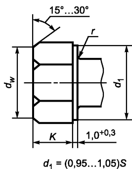
Исполнение 3 головки болта
