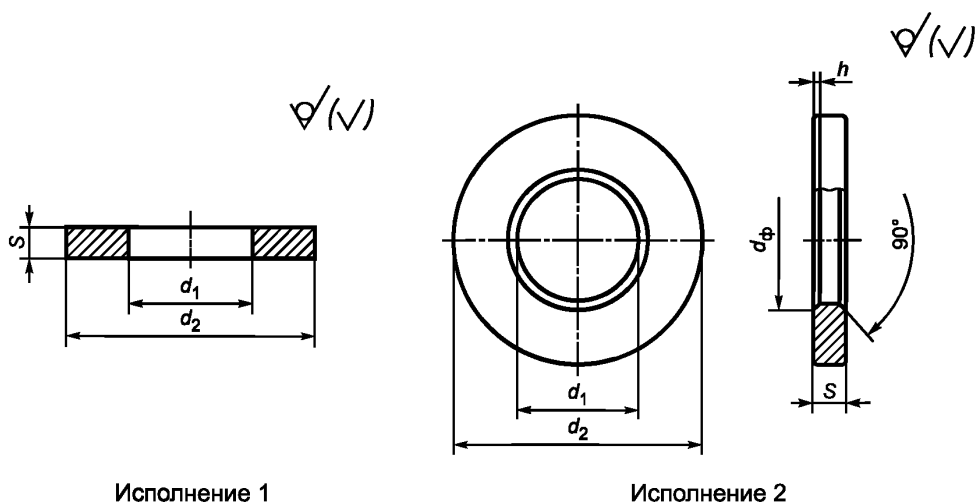
Рисунок 4 — Конструкция шайб
