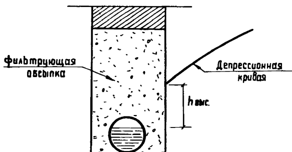
Рис. 20. Расчет высоты высачивания воды
