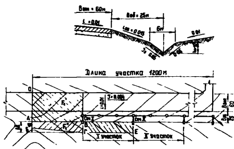
Рис. 3. Расчет коллектора водоотводной сети ИВПИ с лотками на грунтовой поверхности
