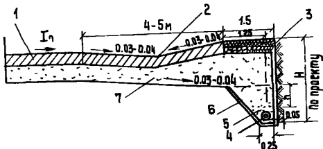
Рис. 11. Вариант конструкции закрочных дрен: 1 - аэродромное покрытие; 2 - лоток в кромке покрытия глубиной 8-10 см; 3 - отмостка; 4 - дренажная труба с внутренним диаметром D_{\text{вн}} = 75-100 мм; 5 - фильтрующая засыпка из крупнозернистого песка; 6 - слой мха или очесов 2-3 см в плотном теле; 7 - песчаное основание
