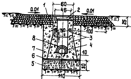
Рис. 9. Конструкция тальвежного колодца: 1 - щебеночная отмостка с пропиткой битумом на 6-8 см; 2 - решетка; 3 - стенка колодца; 4 - перепуск; 5 - шлаковая подушка; 6 - слой цементного раствора; 7 - водостойчивый грунт; 8 - прокладка из просмоленной
