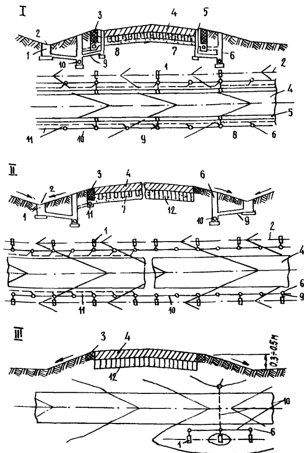
Рис. 4. Схемы водоотводных и дренажных систем (профиль и план) асфальтовых покрытий: I - гальвезный колодец; 2 - грунтовый лоток; 3 - отмостка; 4 - покрытие; 5 - лоток в кромке покрытия; 6 - смотровой колодец; 7 - основание с дренирующим слоем; 8 - дождеприемный колодец; 9 - перепуск; 10 - коллектор; II - закрывчатая дрена; 12 - основание без дренирующего слоя
