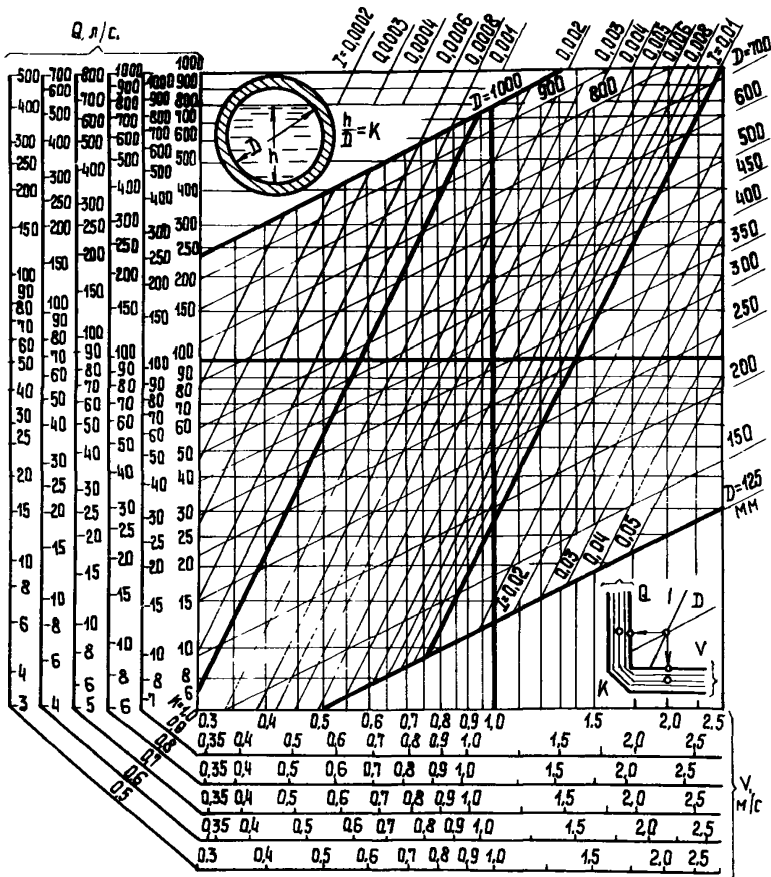
Рис. 6. Номограмма для определения диаметра труб
