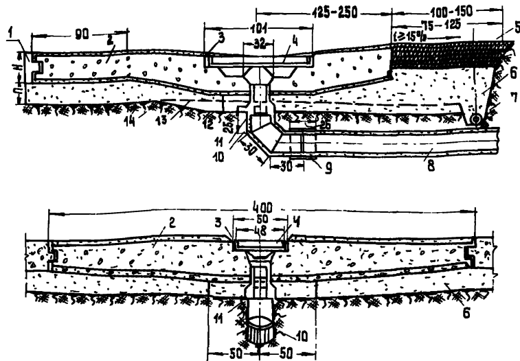
Рис. 10. Конструкция дождеприемного колодца мелкого заложения (вариант с одной решеткой): 1 - асфальтное покрытие; 2 - железобетонная лотковая плита; 3 - заделка щелей цементным раствором состава 1:3; 4 - решетка; 5 - отмостка из щебня с пропиткой битумом на 6-8 см; 6 - песчаное основание; 7 - закрывочная дрена; 8 - перепуск; 9 - стыковая муфта; 10 - сварное колено из стальных труб с антикоррозийной обмазкой; II - прокладка из просмоленной пеньки; 12 - изоляционный слой из битумной мастики; 13 - поверхность дна корыта под лотковыми плитами без дождеприемников; 14 - поверхность дна корыта под плитами с дождеприемными воронками
