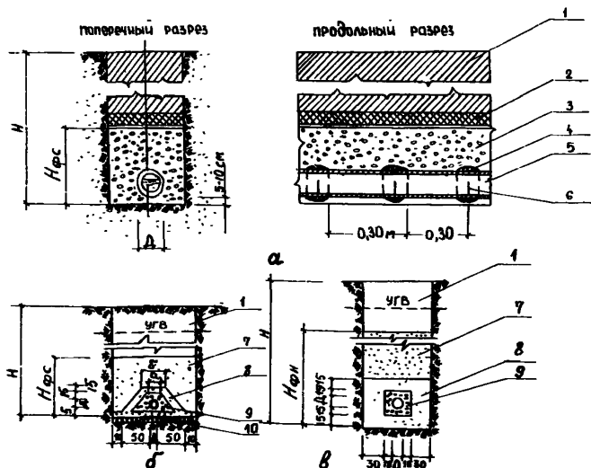
Рис. 12. Варианты конструкций глубинных дрен: а и б - дрена совершенного типа; в - дрена несовершенного типа; 1 - местный грунт; 2 - древесина; 3 - фильтрующая засыпка; 4 - слой мха, очесы или минеральная вата; 5 - труба асбестоцементная D = 100 мм; 6 - шель (пропил) в трубе; 7 - песок с коэффициентом фильтрации не менее 7 м/сут.; 8 - песок; 9 - щебень; 10 - щебень, втрамбованный в грунт
