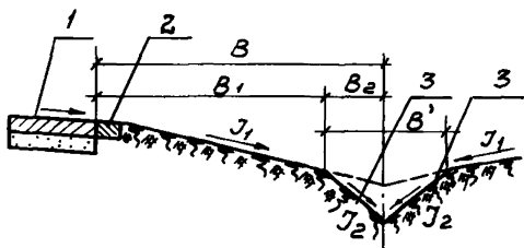
Рис. 7. Схема устройства "лотка в лотке": 1 - аэродромное покрытие; 2 - отмостка; 3 - лоток в лотке
