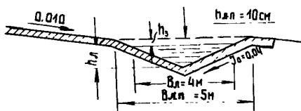
Рис. 2. Расчет лотка треугольного сечения
