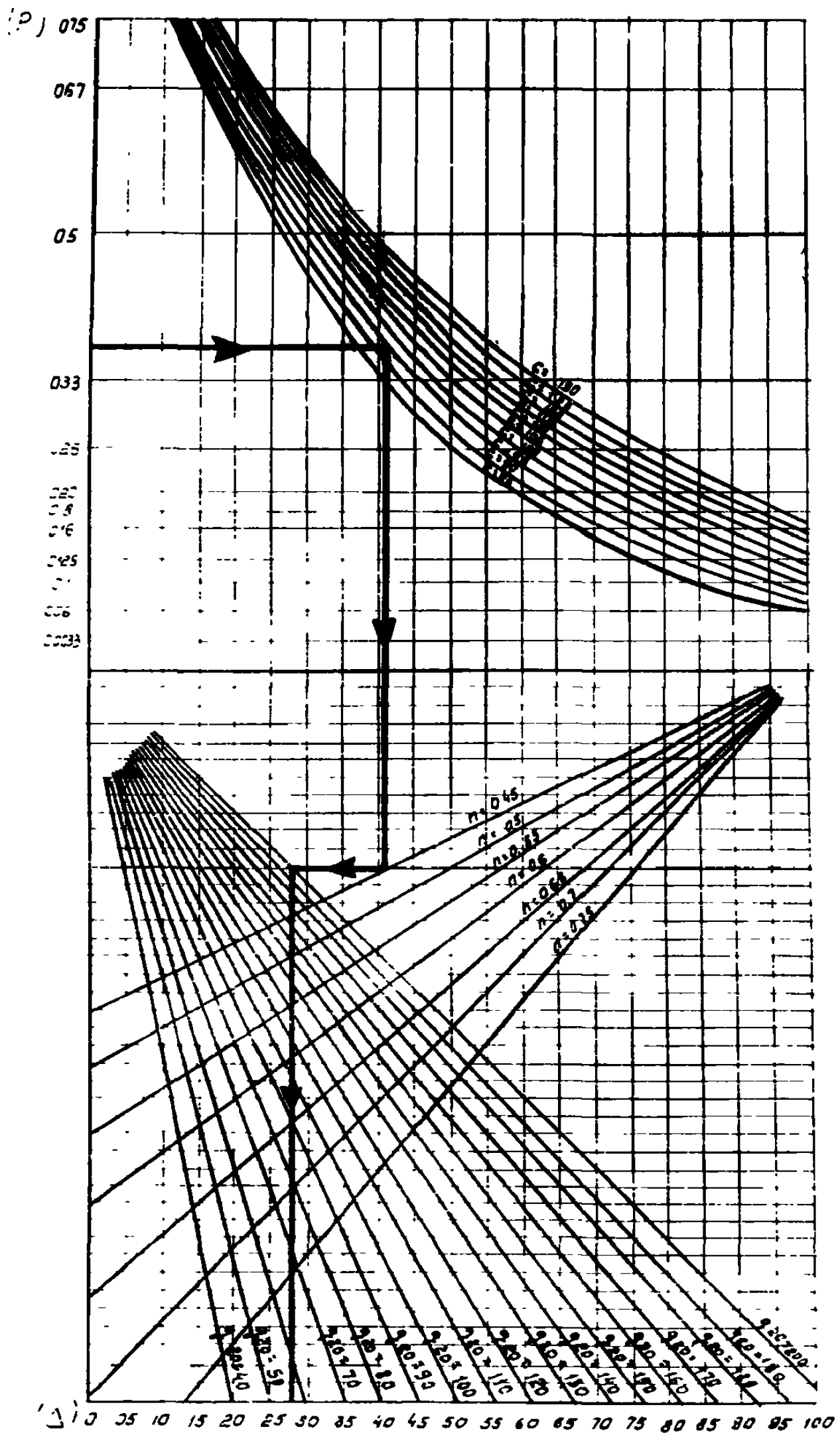
Рис. 2. Номограммы для определения параметра \Delta
