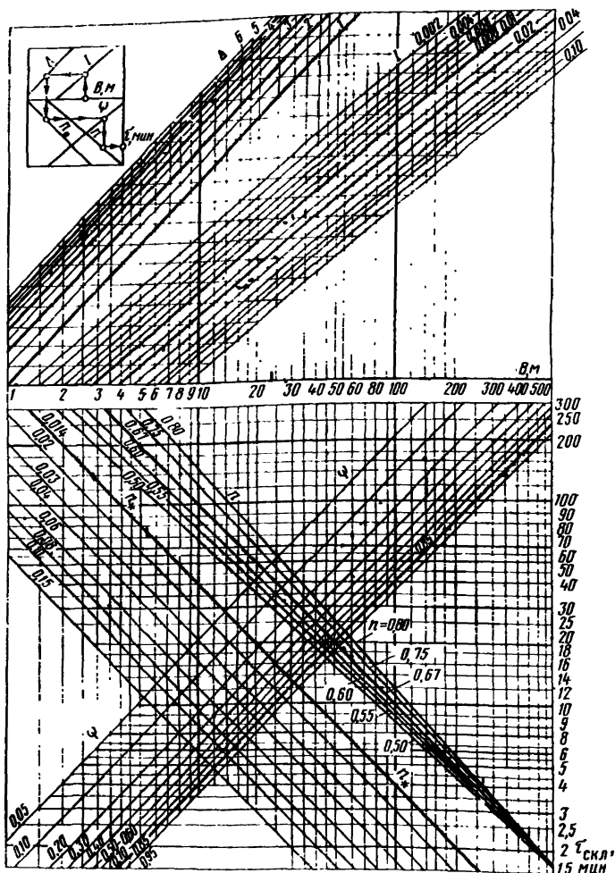
Рис. 3. Номограмма для определения времени добегаания дождевых вод по склону I_{\text{скл}} : V — длина стока; I — уклон стока; K^* — коэффициент шероховатости поверхности; \Psi — коэффициент стока; \Delta — интенсивность одноминутного дождя; n — показатель степени
