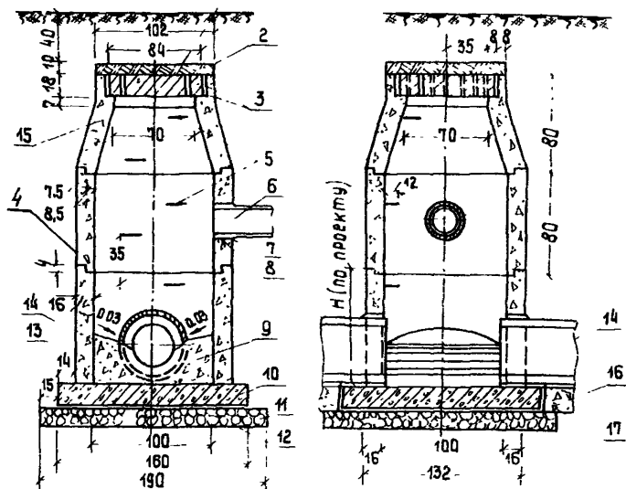
Рис. 15. Конструкция круглого смотрового колодца с заглубленной крышкой (сборный из железобетонных звеньев): 1 - крышка; 2 - заделка мягкой глиной слоем 10 см; 3 - отверстия 18x6x2 см; 4 - среднее бетонное кольцо с гнездом для перепуска; 5 - скобы \varnothing 16 мм; 6 - перепуск; 7 - битум; 8 - просмоленная пенка \delta = 1, 0-1,5 см; 9 - бетонный лоток (набивается на месте); 10 - железобетонное дно; 11 - щебеночная подготовка; 12 - цементный раствор; 13 - нижнее бетонное кольцо (бетонируется на месте); 14 - труба коллектора; 15 - горловина; 16 - сборное основание под трубу; 17 - температурный шов \delta = 2 см
