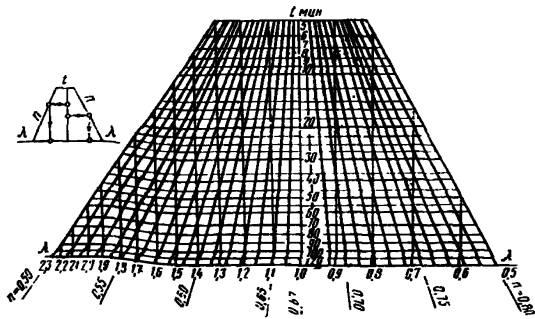
Рис. 1. Номограмма для определения величины поверхностного стока S : а - для цементобетонных покрытий ( \rho = 0,85 и n = 0,67 ); б - для определения поправки \lambda к величине S в случае значений n \neq 0,67
