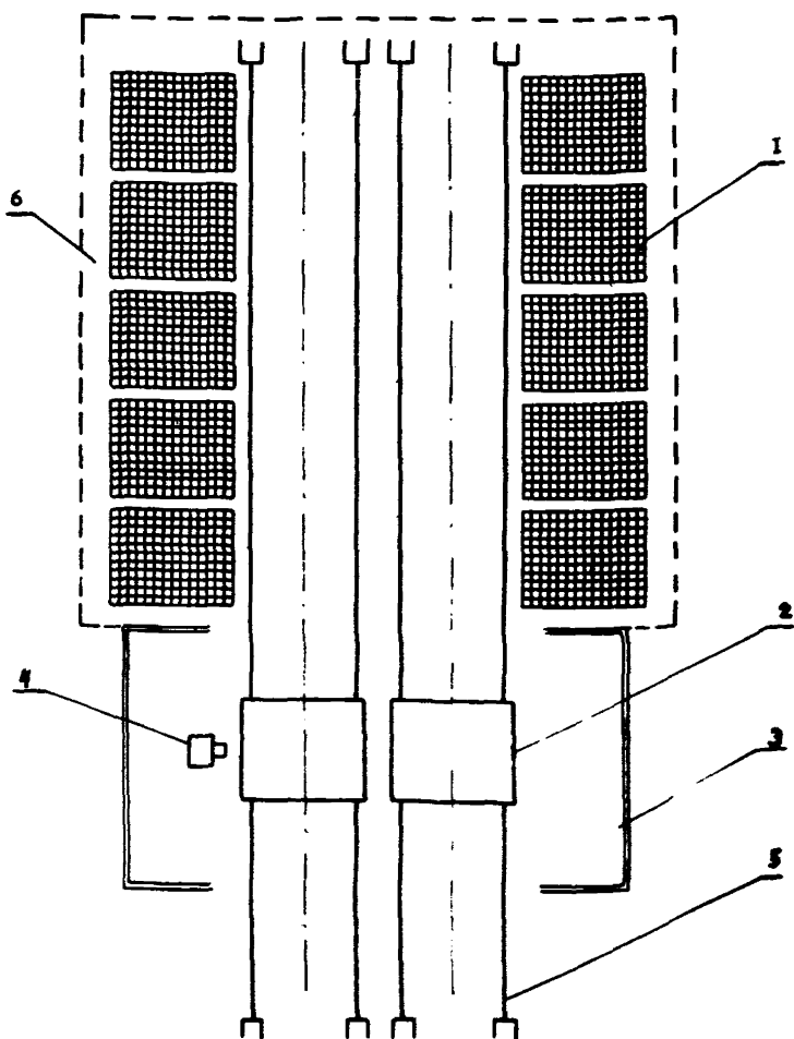
Рис.1. Схема арматурного цеха с подвижными кондукторами: 1-штабеля готовой арматурной сетки; 2-подвижные кондукторы; 3-арматурный цех; 4-подвесные вешки для контактной сварки К-260; 5-рельсы; 6-склад готовой продукции
