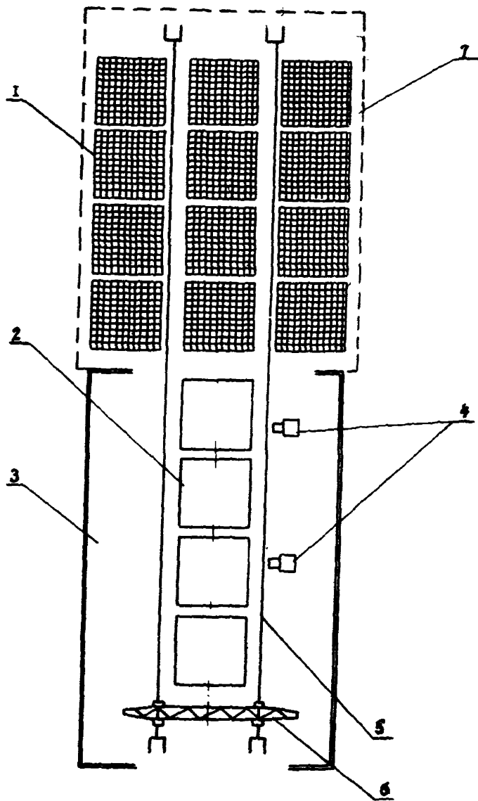
Рис.2. Схема арматурного цеха с неподвижными кондукторами: 1-штабеля готовой арматурной сетки; 2-кондукторы; 3-арма - турный цех; 4-подвесная машина для контактной сварки МТПП-75-1 с клешнями КТП-1; 5-подкрановые пути; 6-козловой кран К-4М; 7-склад готовой продукции
