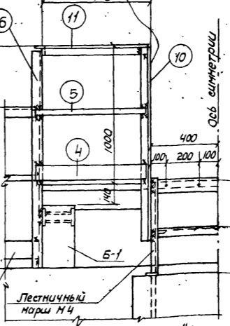
Вид по Б
