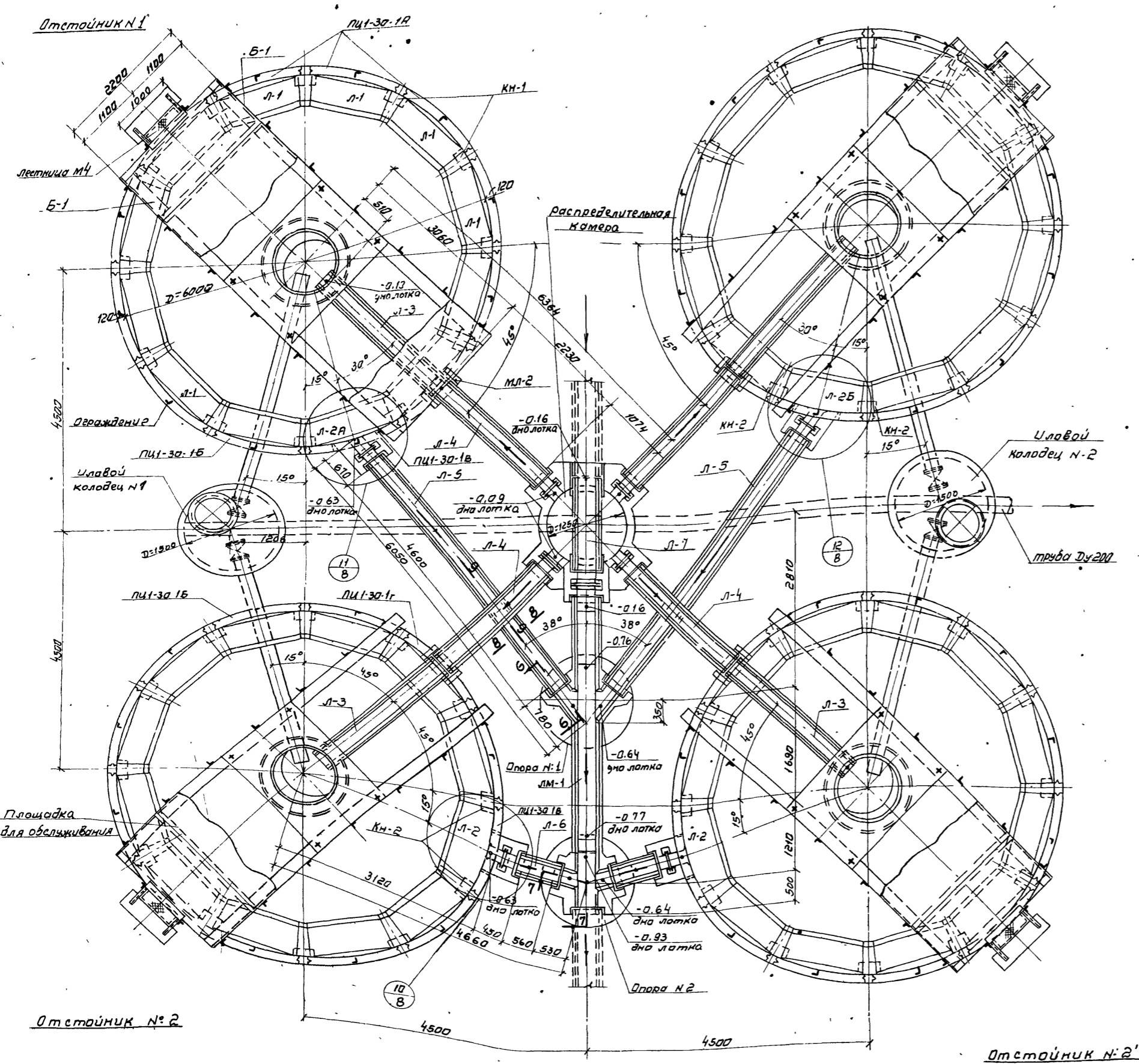
Отстойник № 1
