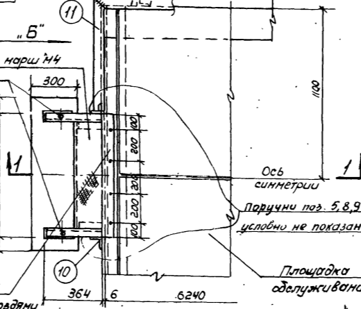
План по 2-2
