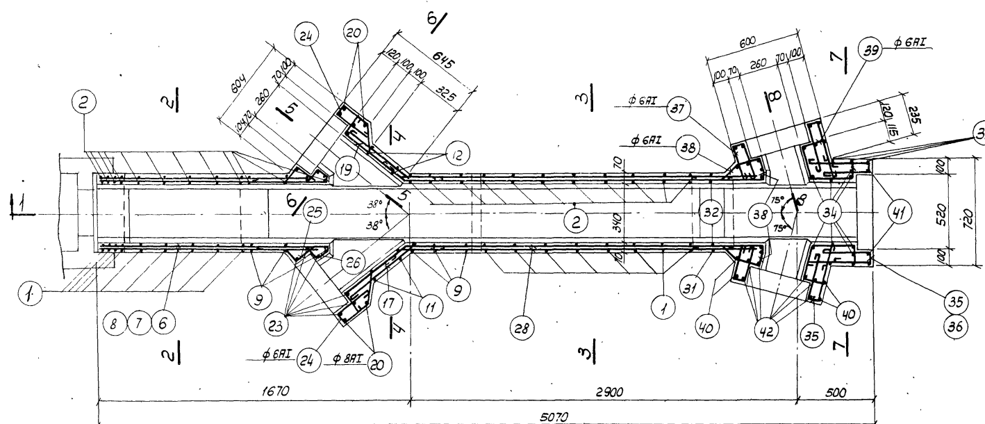
План
