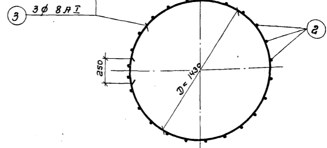
Развертка сетки С-2
