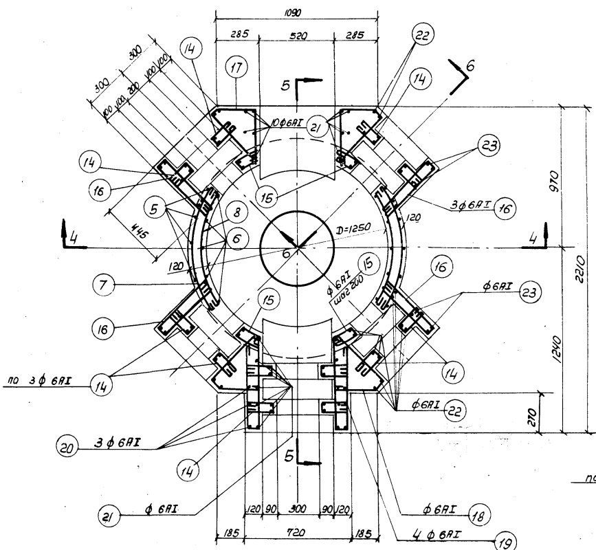
План 1-1
