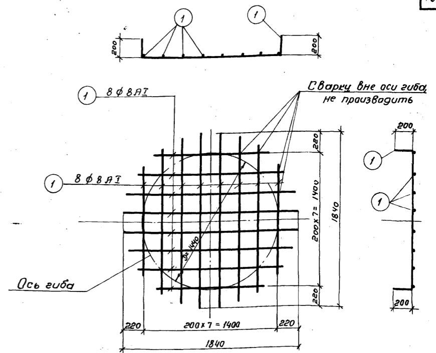
Сетка С-1
