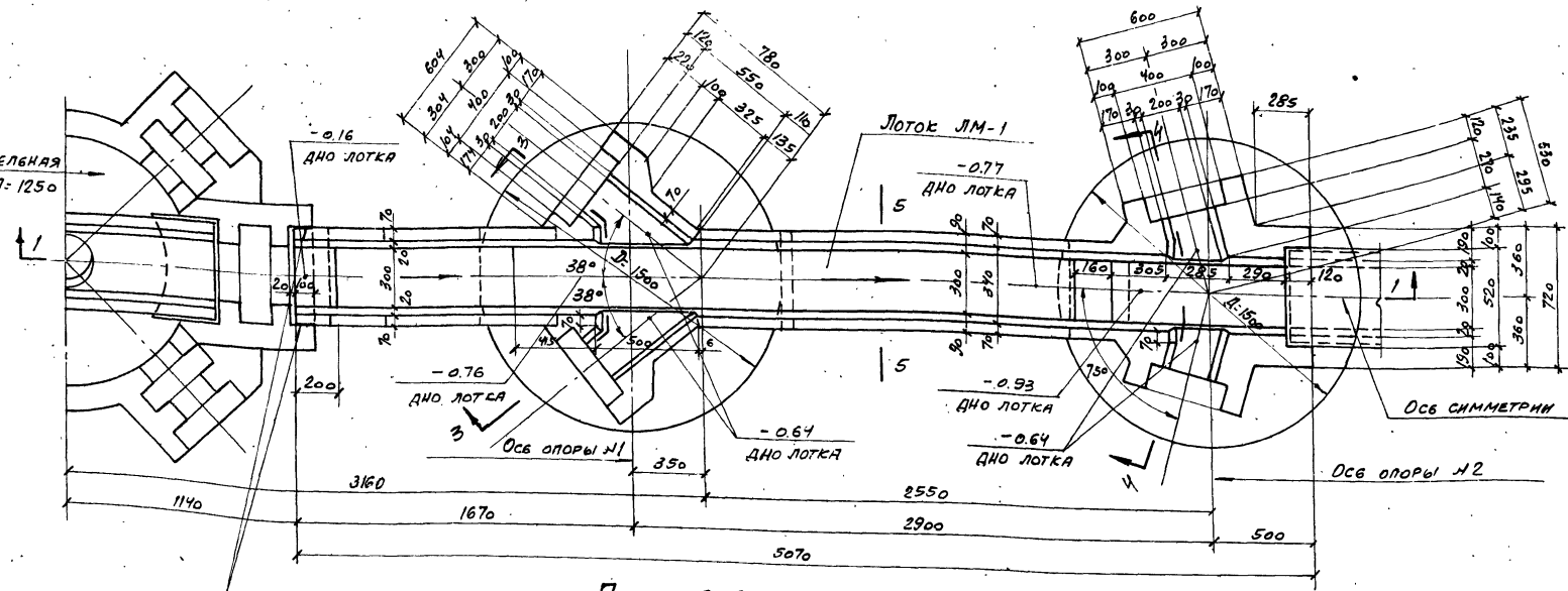
ПЛАН 2-2
