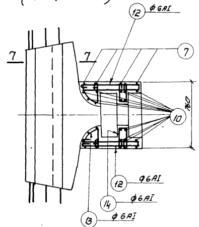
План Б-Б для Л-2 (армирование)
