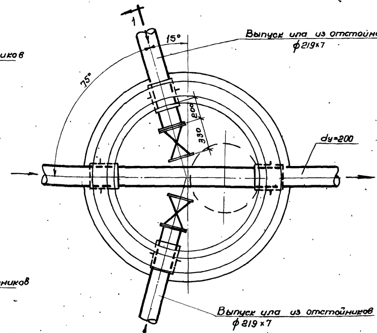
План 2-2 Щловой колодец №2
