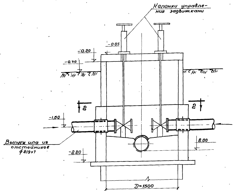
Разрез 1-1
