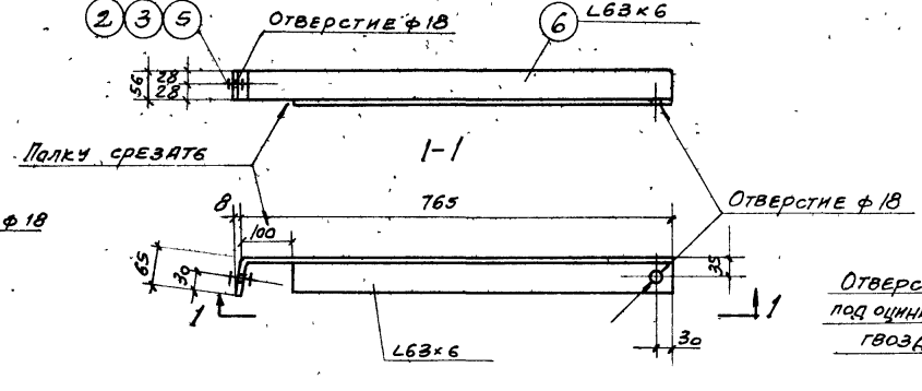
M-3T (M-3H ИЗГОТОВИТЬ НАОБОРОТ) СМ. ЛИСТ АС-6
