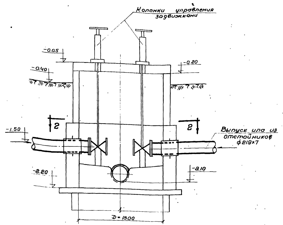
Разрез 1-1
