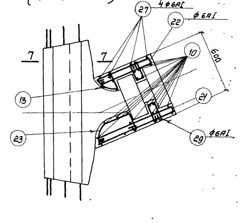
План Г-Г для Л-2А (армирование лотка Л-2Б аналогично лотку Л-2А)
