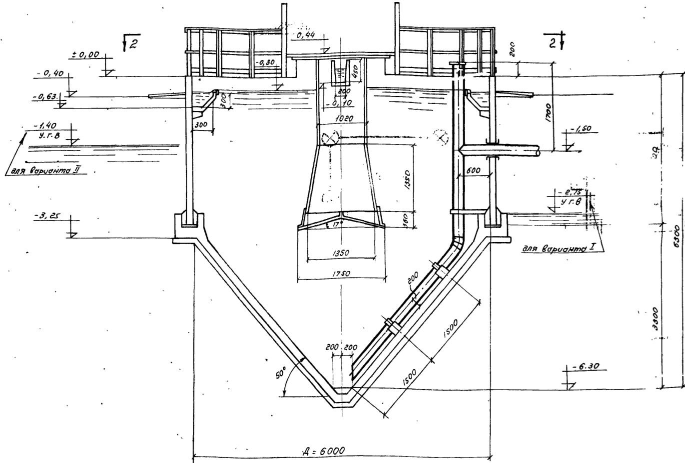
разрез 1-1
