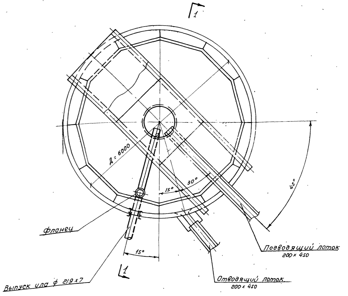
План 2-2
