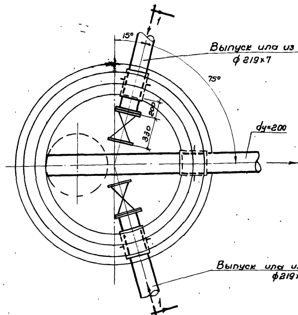
План 2-2 Щловой колодец №1
