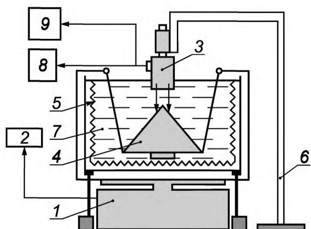
Рисунок F.2 — Компоновка В с выпуклой отражающей мишенью:
