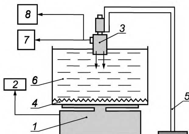
Рисунок F.4 — Компоновка С с поглощающей мишенью:
