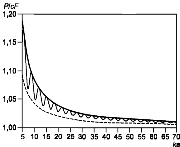
Рисунок Е.1 — Зависимость P/cF от ka (осциллирующая кривая) с аппроксимацией «по пикам» (сплошная линия) и центральной (по половинным значениям) линий (пунктирная кривая), представляющей поправочный коэффициент corr
