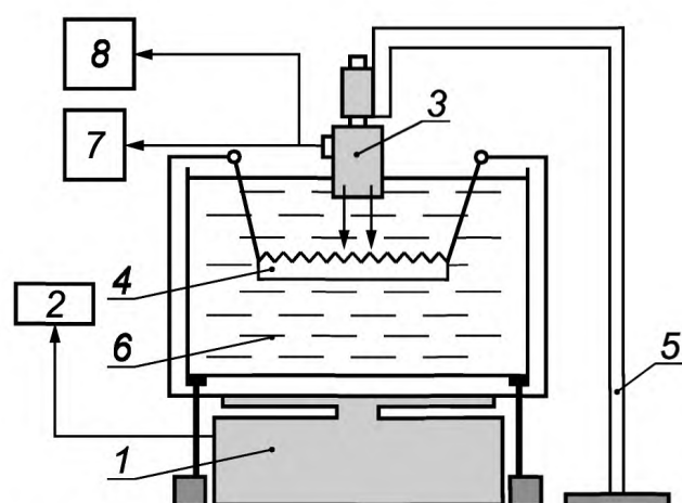
Рисунок F.3 — Компоновка В с поглощающей мишенью:
