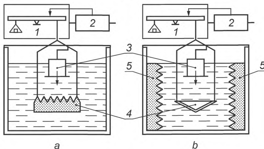
Рисунок F.5 — Компоновка Е с поглощающей (а) и вогнутой отражающей (b) мишенями:
