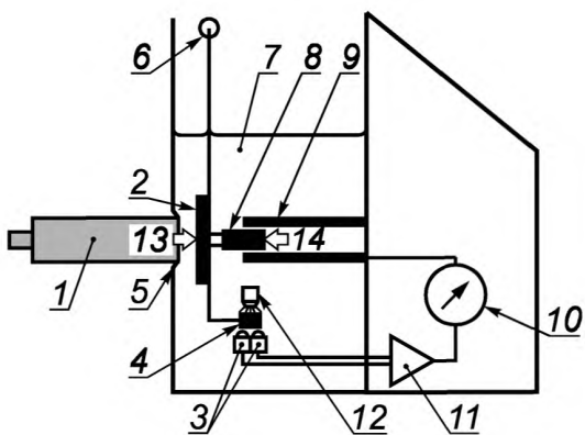
Рисунок F.7 — Компоновка F с поглощающей мишенью:
