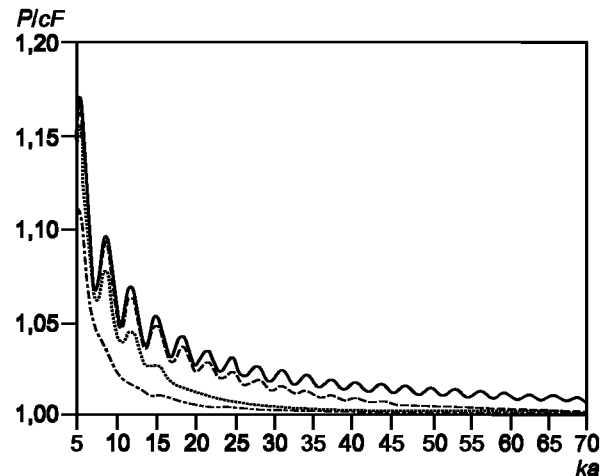
Рисунок Е.2 — Зависимость P/cF от ka для четырех различных псевдотрапецевидных амплитудных распределений: для \varepsilon = 0 (поршень) (сплошная кривая), \varepsilon = 0,1 (штриховая), \varepsilon = 0,25 (точечная), \varepsilon = 0,6 (штрихпунктирная)
