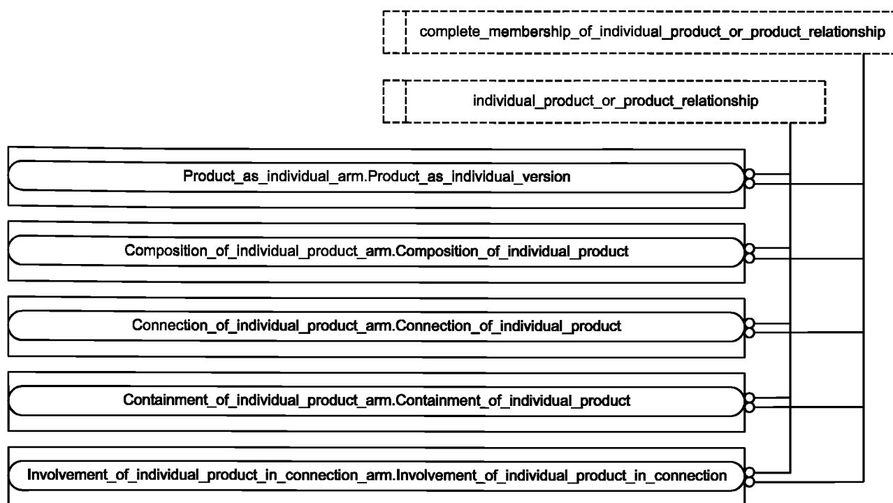
Рисунок С.2 — Представление ПЭМ на уровне объектов в формате EXPRESS-G (диаграмма 1 из 2)
