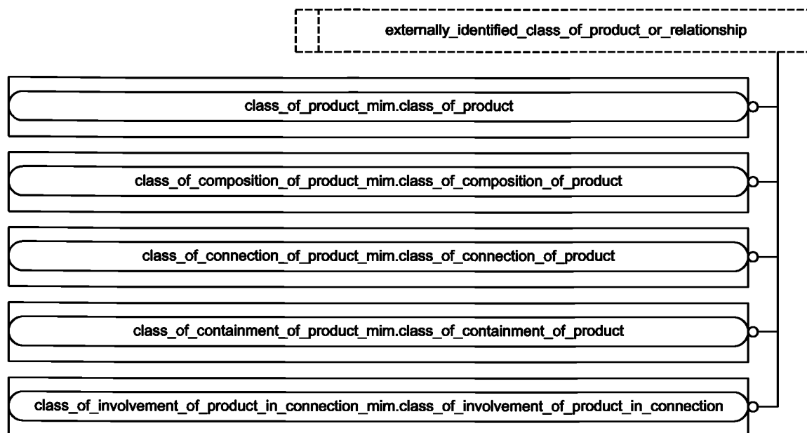
Рисунок D.3 — Представление ИММ на уровне объектов в формате EXPRESS-G (диаграмма 2 из 2)
