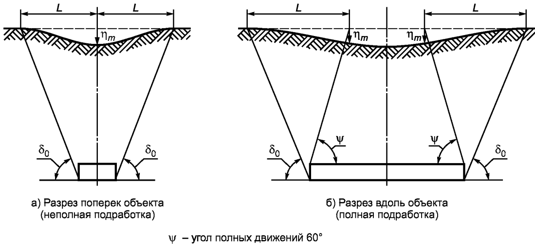
Рисунок С.1 — Основные параметры мульды сдвижения
