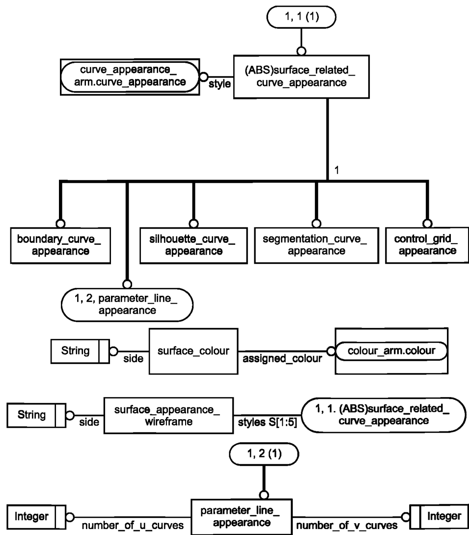
Рисунок С.1 — EXPRESS-G диаграмма ПЭМ
