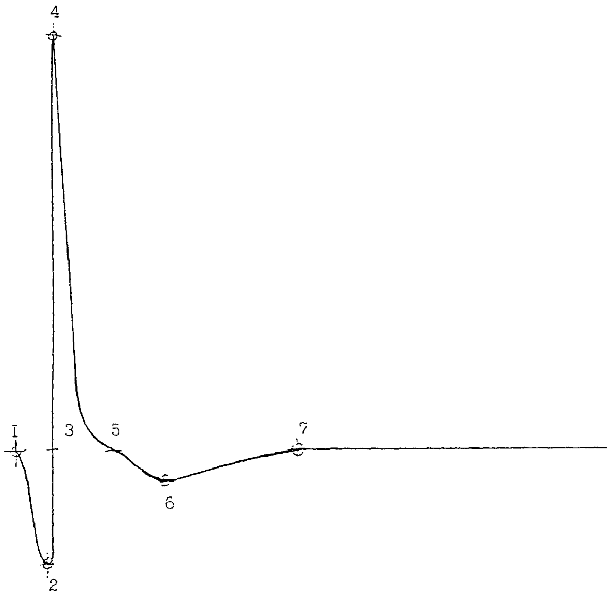
Рисунок А.2 - форма сигнала "ЭМГ-2" (ПЗУ "М2") (к таблице А.1).
