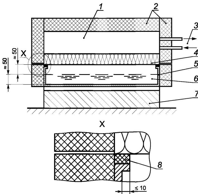
1 — охлаждающая пластина; 2 — теплоизоляция охлаждающей пластины и контейнера; 3 — вход и выход для охлаждающего реагента; 4 — образец; 5 — коррозионно-стойкий контейнер с рамой, поддерживающей образец; 6 — водопроводная вода; 7 — нагревательное устройство с термостатом; 8 — герметик
