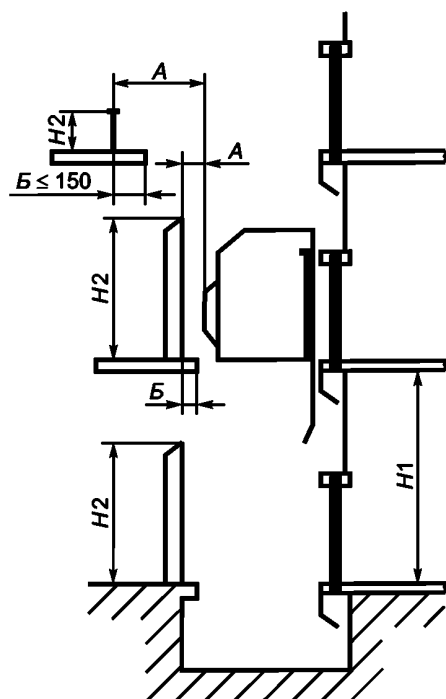
А — расстояние до движущихся элементов лифта; В — расстояние между ограждением и краем межэтажных перекрытий, ступеней и площадок; H1 — высота ограждения со стороны этажной площадки; H2 — высота ограждения с остальных сторон
