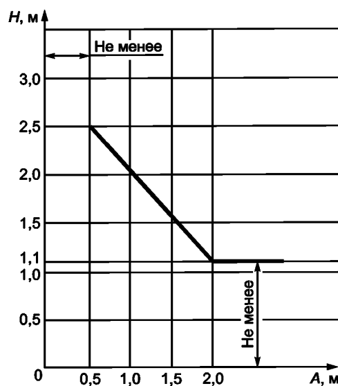
А — расстояние от движущихся элементов лифта; H — высота ограждения
