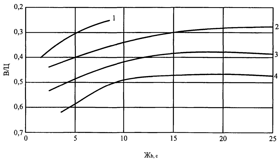
Рис.1. Графики для подбора отношения Ц:П, обеспечивающего требуемую жесткость сталефибробетонной смеси в зависимости: а – от жесткости исходного бетона при \mu_{fv} : 1-1%; 2-1,5%; 3-2,5%. б – цементно-песчаного отношения Ц:П от жесткости исходного бетона Ж_{б,с} и водоцементного отношения Ц:П равного: 1-1:1; 2-1:2; 3-1:3; 4-1:4.
