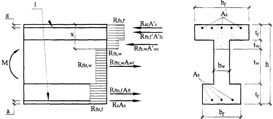
Рисунок 6.3 - Схема распределения усилий и эпюра напряжений в сечениях, нормальных к продольной оси изгибаемого элемента двутаврового сечения при комбинированном армировании
