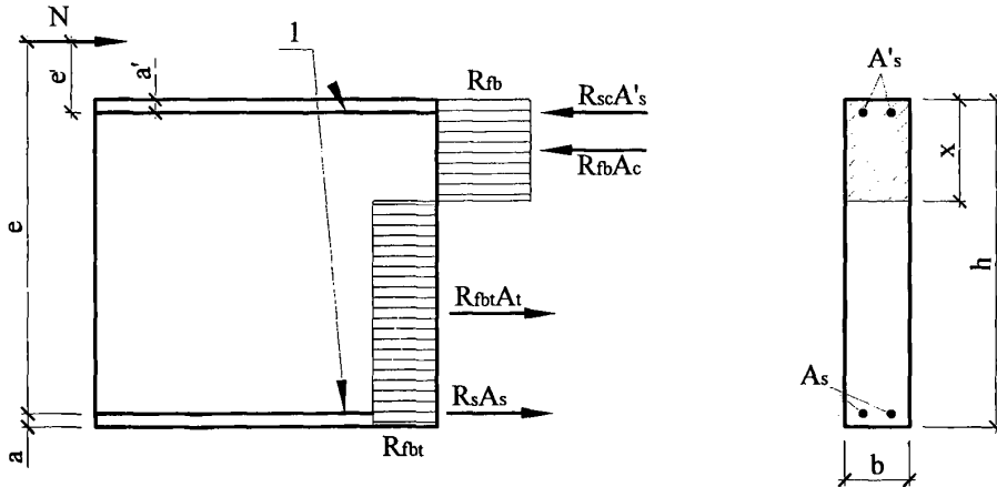
Рисунок 6.5 - Схема усилий и эпюра напряжений в сечении, нормальном к продольной оси сжатого сталефибробетонного элемента, при его расчете по прочности (при комбинированном армировании) 1 – стержневая арматура
