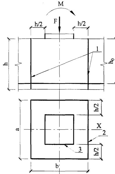
Рисунок 6.13 – Схема для расчета сталефибробетонных элементов без поперечной арматуры на продавливание;
