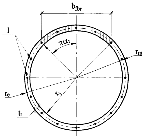
Рисунок 6.4 - Схема кольцевого сечения сталефибробетонного элемента, принимаемая при его расчете по прочности на изгиб (при комбинированном армировании) 1 – стержневая арматура
