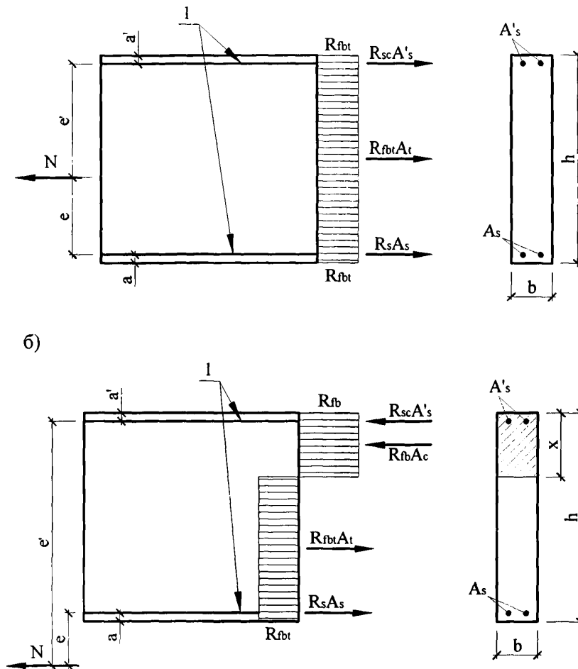
Рисунок 6.8 - Схема усилий и эпюра напряжений в сечении, нормальном к продольной оси внецентренно растянутого сталефибробетонного элемента, при его расчете по прочности, при приложении продольной силы N : а) между равнодействующими усилий в арматуре S и S' ; б) за пределами расстояния между равнодействующими усилий в арматуре S и S' 1 – стержневая арматура
