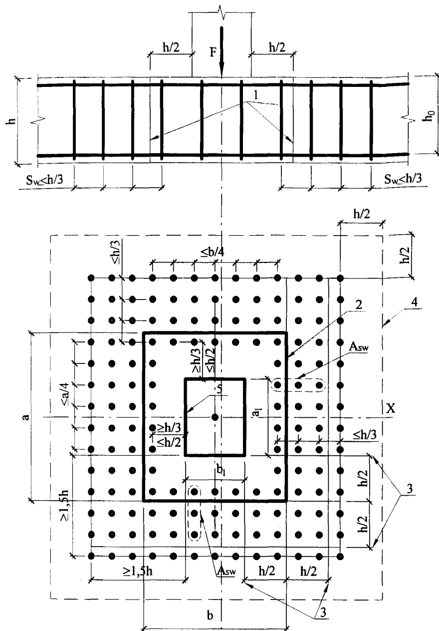
Рисунок 6.14 – Схема для расчета сталефибробетонных плит с вертикальной равномерно распределенной поперечной арматурой на продавливание:
