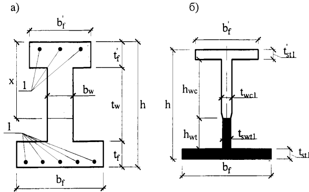
Рисунок 7.1 - Схема приведения сечения сталефибробетонных элементов к стальному: а) сечение сталефибробетонного элемента; б) сечение, приведенное к стальному; 1- стержневая арматура.
