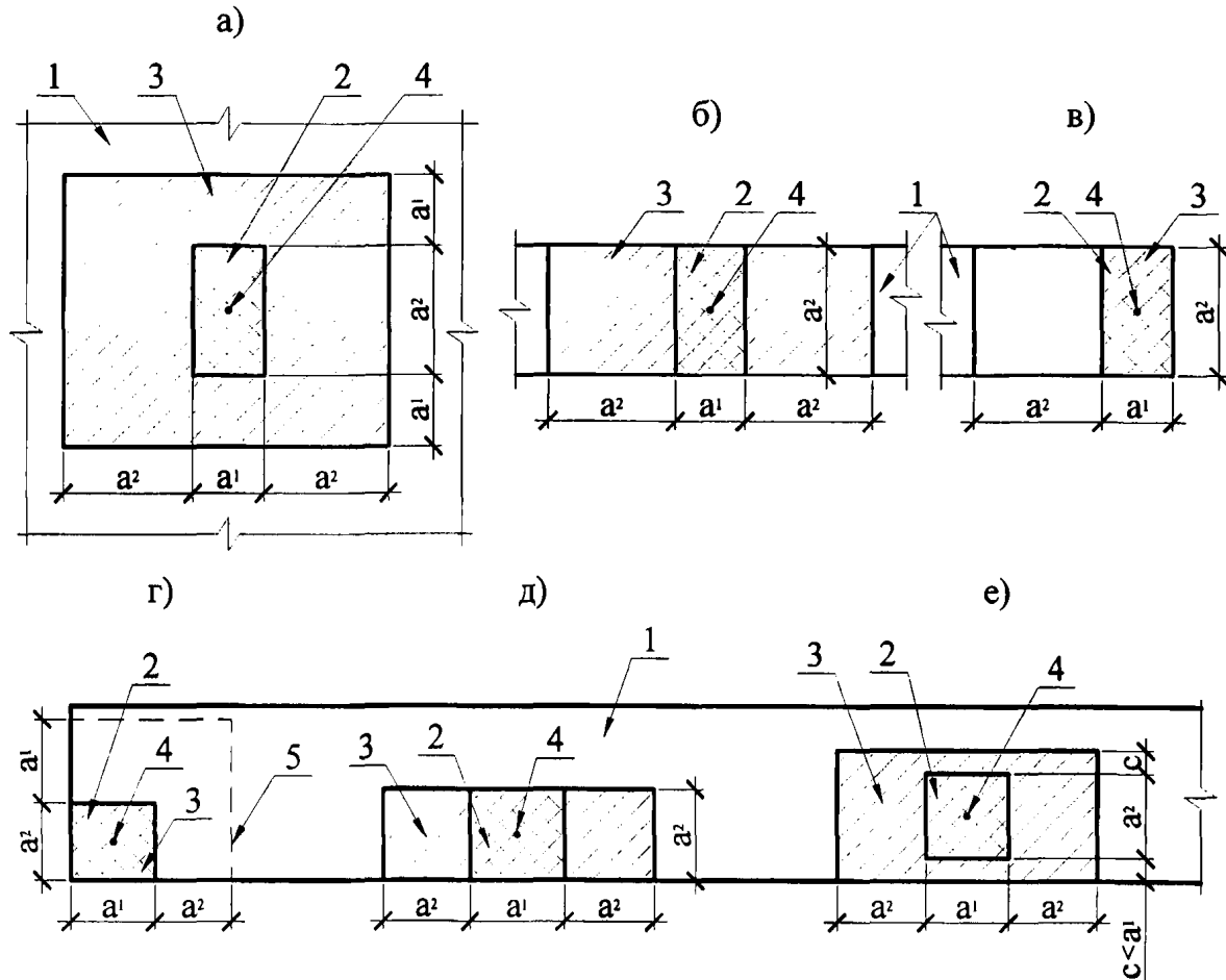
Рисунок 6.11 – Схемы для расчета элементов на местное сжатие при расположении местной нагрузки: а) – вдали от краев элемента; б) – по всей ширине элемента; в) – у края (торца) элемента по всей его ширине; г) – на углу элемента; д) – у одного края элемента; е) – вблизи одного края элемента. 1 – элемент, на который действует местная нагрузка; 2 – площадь смятия A_{fb,loc} ; 3 – максимальная расчетная площадь A_{fb,max} ; 4 – центр тяжести площадей A_{fb,loc} и A_{fb,max} ; 5 – минимальная зона армирования сетками, при которой косвенное армирование учитывается в расчете.
