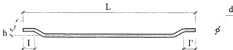
Рис.1 Форма и размеры фибры типа «ФЛА»
