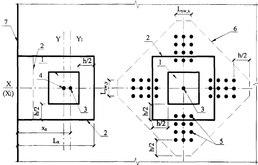
Рисунок 6.12 – Схема расчетных контуров поперечного сечения при продавливании: а, в) – площадка приложения нагрузки у края плоского элемента; б) – то же внутри плоского элемента; г) – при крестообразном расположении поперечной арматуры. 1 – площадь приложения нагрузки; 2 – расчетный контур поперечного сечения; 2' – второй вариант расположения расчетного контура; 3 – центр тяжести расчетного контура (место пересечения осей X_1 и Y_1 ); 4 – центр тяжести площадки приложения нагрузки (место пересечения осей X и Y ); 5 – поперечная арматура; 6 – контур расчетного поперечного сечения без учета в расчете поперечной арматуры; 7 – граница (край) плоского элемента.
