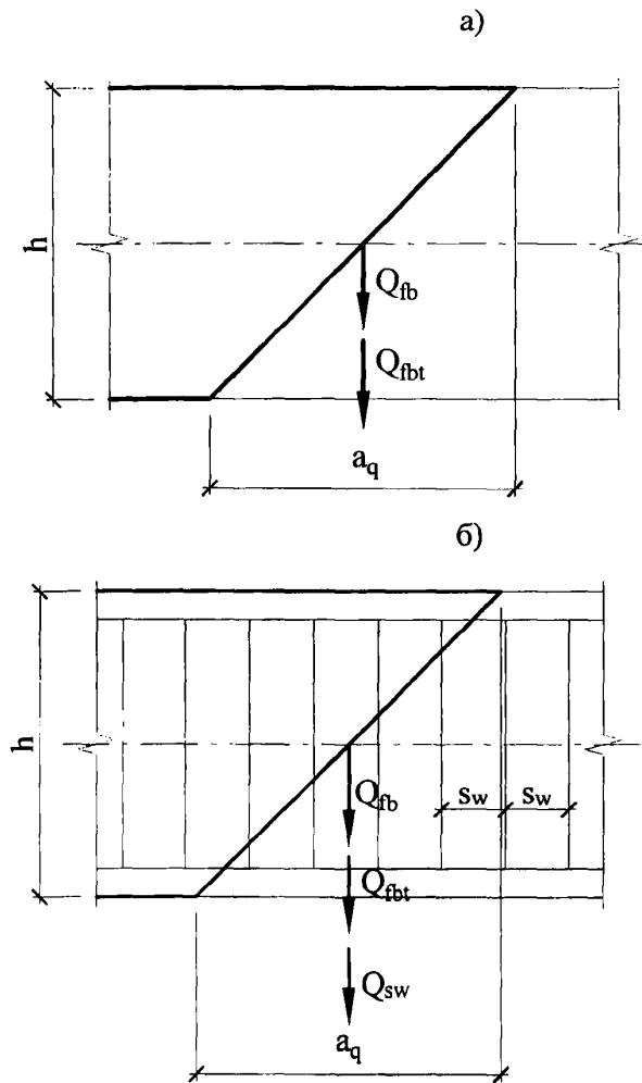
Рисунок 6.9 - Схема усилий при расчете сталефибробетонных элементов по наклонному сечению на действие поперечных сил: а) при фибровом армировании; б) при комбинированном армировании.
