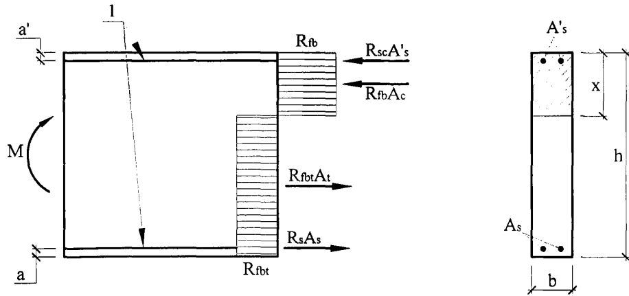
Рисунок 6.2 - Схема усилий и эпюра напряжений в сечении, нормальном к продольной оси изгибаемого сталефибробетонного элемента прямоугольного сечения, при его расчете по прочности (при комбинированном армировании) 1 – стержневая арматура
