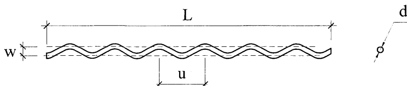
Рис.2 Форма и размеры фибры типа «ФВ»
