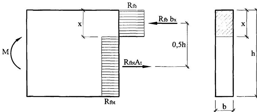
Рисунок 6.1 - Схема усилий и эпюра напряжений в сечении, нормальном к продольной оси изгибаемого сталефибробетонного элемента прямоугольного сечения, при его расчете по прочности (при фибровом
