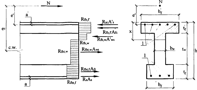
Рисунок 6.6 - Схема усилий и эпюра напряжений во внецентренно сжатых элементах двутаврового сечения при комбинированном армировании:
