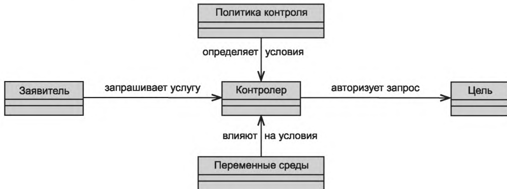
Рисунок 7 — Модель контроля
