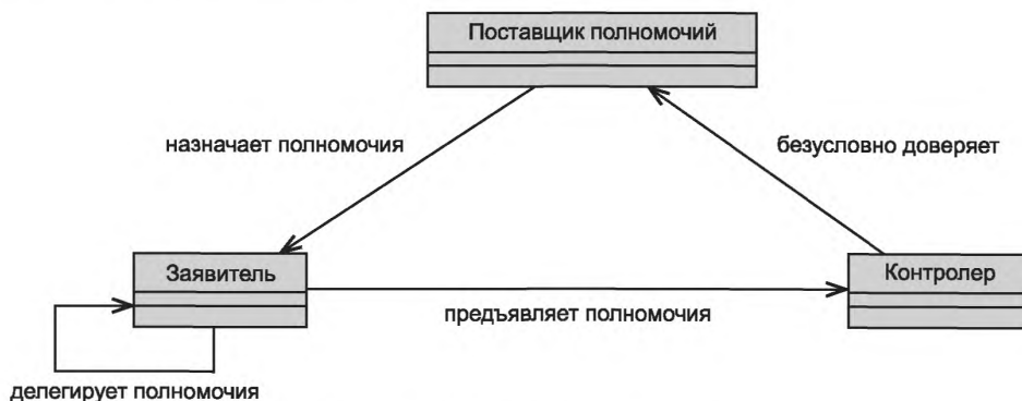
Рисунок 8 — Модель делегирования
