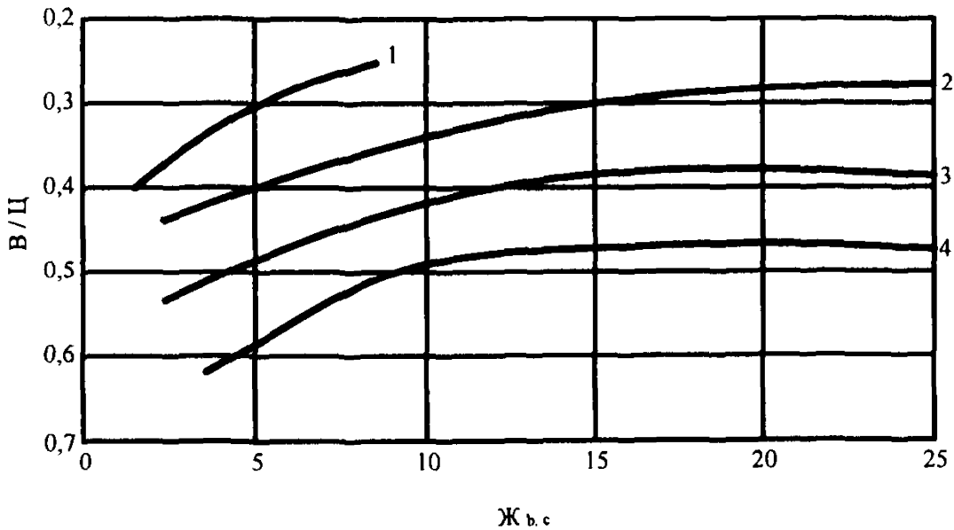
Рис. 1. Графики для подбора отношения Ц:П, обеспечивающего требуемую жесткость сталефибробетонной смеси в зависимости: а – от жесткости исходного бетона при \mu_{fv} : 1-1%; 2-1,5%; 3-2,5%. б – цементно-песчаного отношения Ц:П от жесткости исходного бетона Ж_б и водоцементного отношения Ц:П равного: 1-1:1; 2-1:2; 3-1:3; 4-1:4.
