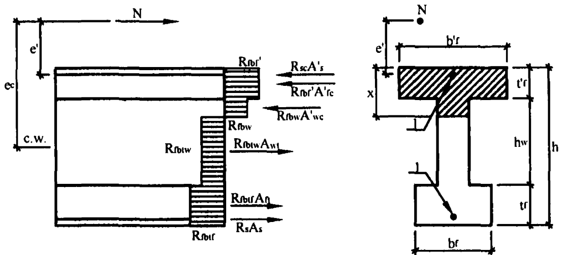
Рис.6. Схема усилий и эпюра напряжений во внецентренно сжатых элементах двутаврового сечения при комбинированном армировании при x > t'_r
