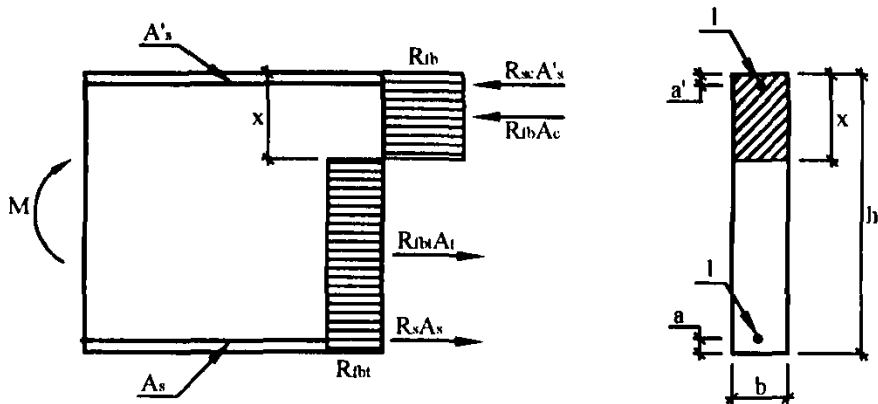
Рис.3. Схема усилий и эпюра напряжений в сечениях, нормальных к продольной оси изгибаемого железобетонного элемента прямоугольного сечения при комбинированном армировании
