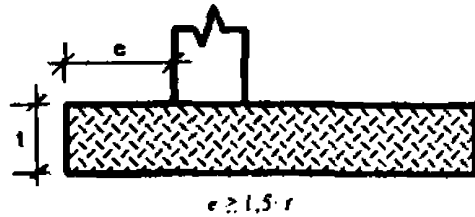
Тип 1. Армирование стальной фиброй
