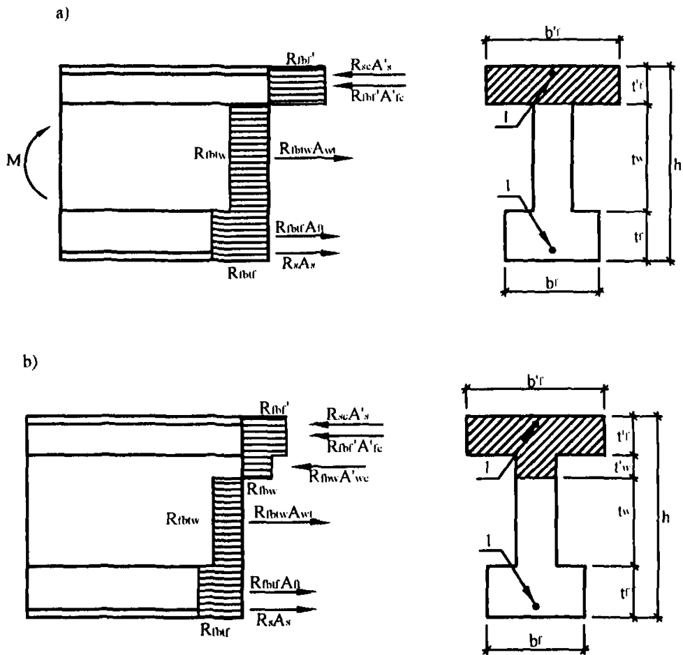
Рис.4. Схема распределения усилий и эпюра напряжений в сечениях, нормальных к продольной оси изгибаемого элемента двутаврового сечения при комбинированном армировании
