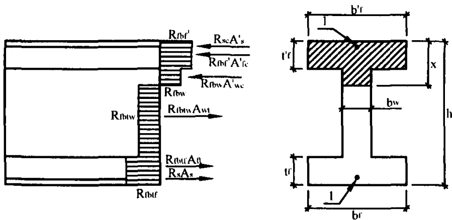
Рис.1. Схема внутренних усилий и эпюры напряжений в сечении, нормальном к продольной оси элемента (общий случай)
