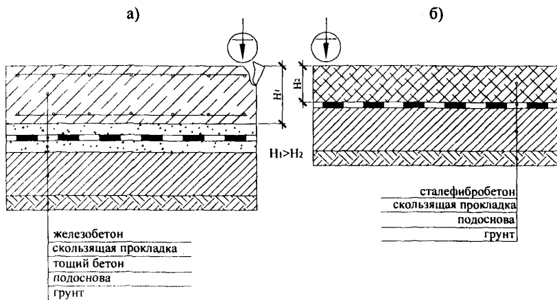
Рис.1. Сопоставительные конструктивные решения промышленных полов по грунтам:
