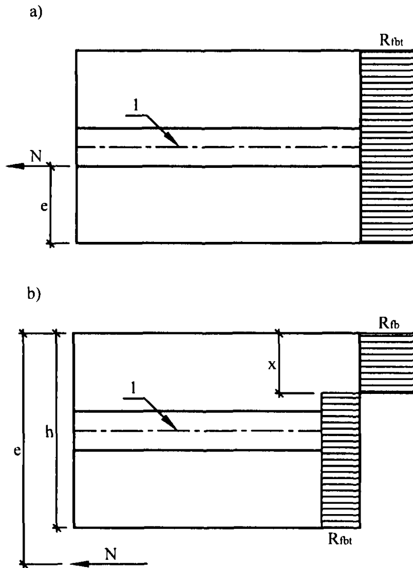
Рис.7. Эпюры напряжений во внецентренно растянутых элементах прямоугольного сечения
