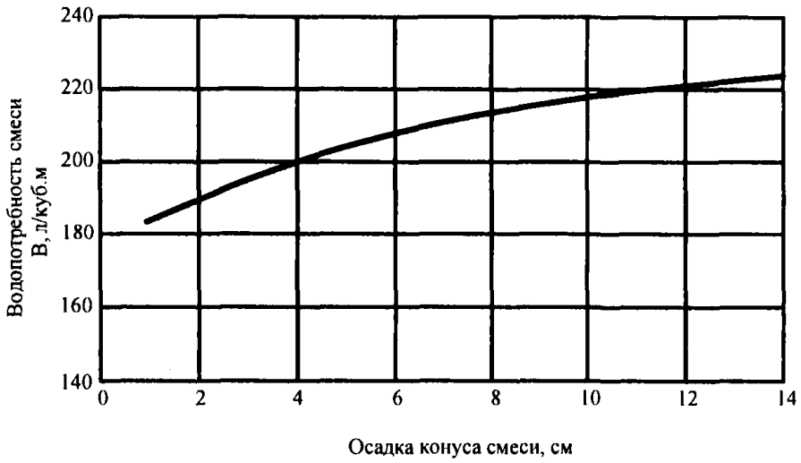
Рис. 3 График водопотребности пластичной (а) и жесткой (б) бетонной смеси
