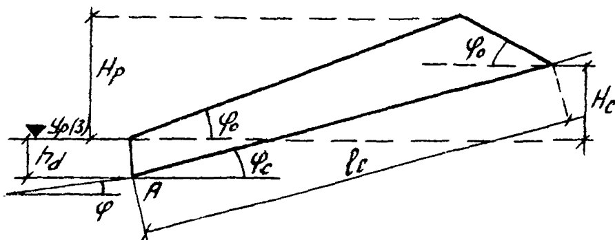
Рис. 3. Расчетная схема надвига льда на откос сооружения
