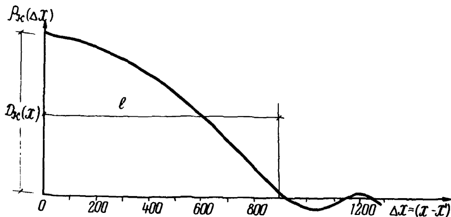
Рис.5. Характерный вид нормированной корреляционной функции стационарной случайной функции R_k(x) :
