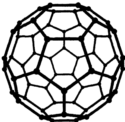
Рис. 1. Структура фуллерена C_{60}
