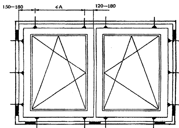
а) Оконный блок с вертикальным импостом
