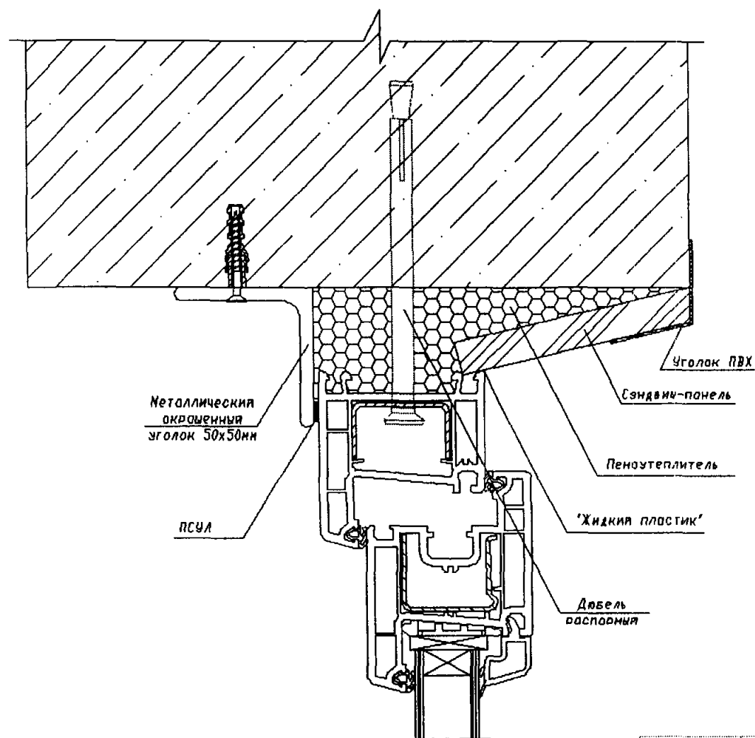
Схема верхнего/бокового узла примыкания ОБ к однослойной бетонной панельной стене.
