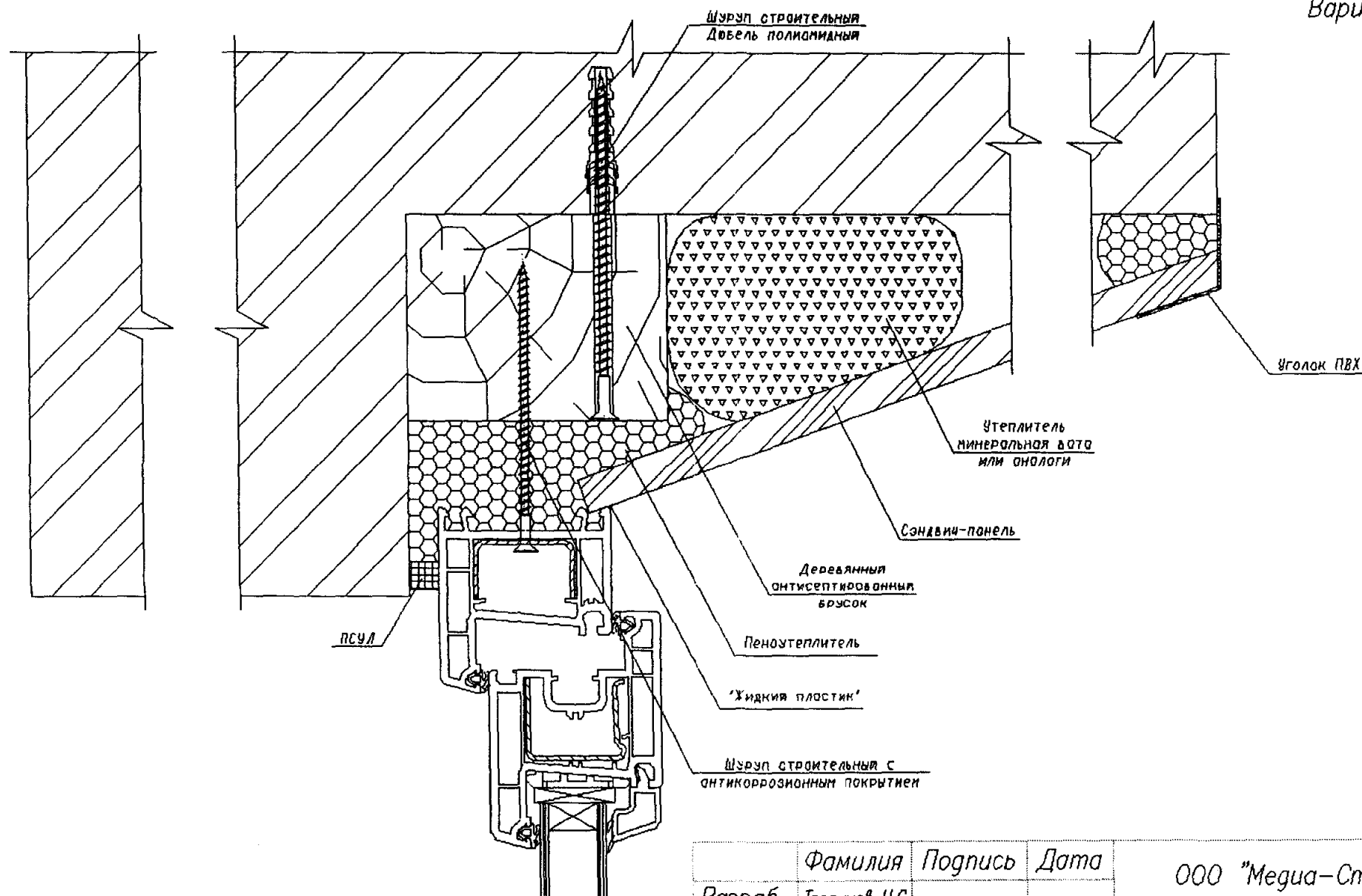
Схема верхнего/бокового узла примыкания ОБ к кирпичной стене "старого фонда".
