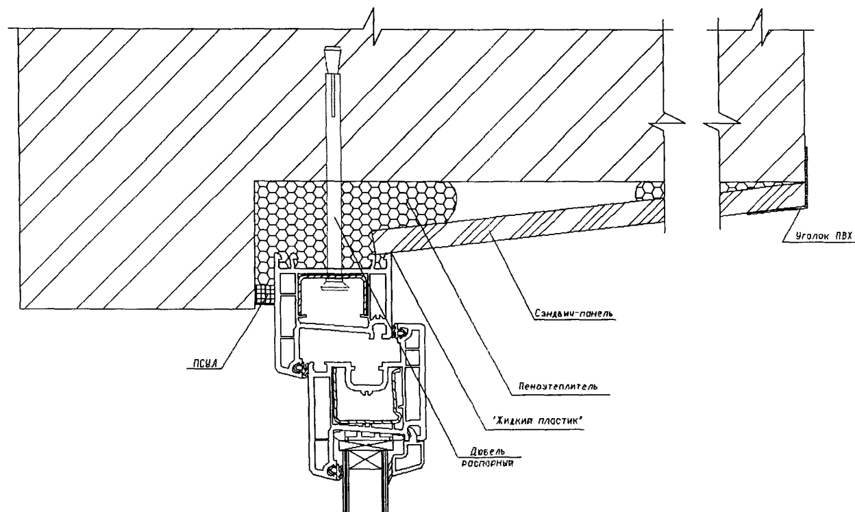
Схема Верхнего/бокового узла примыкания ОБ к кирпичной стене с четвертью.
