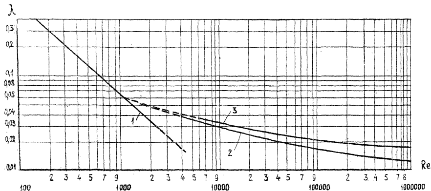
ГРАФИК ЗАВИСИМОСТИ \lambda ОТ КРИТЕРИЯ Re
