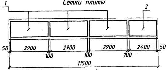
Схема расположения сеток Сетки плиты
