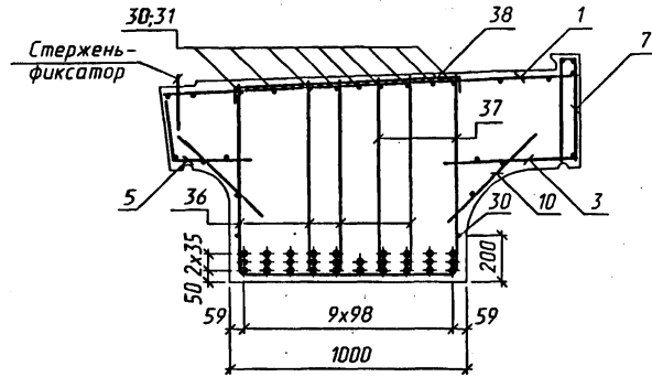
Сечение в середине пролета
