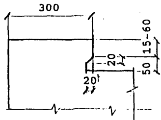
Деталь заделки изоляции 1:10
