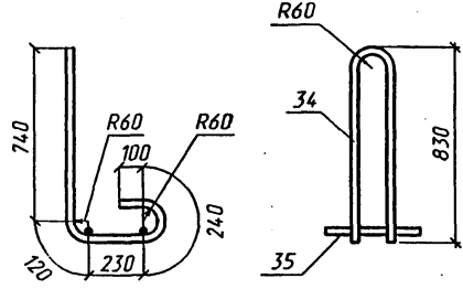
Деталь заделки строповочной петли
