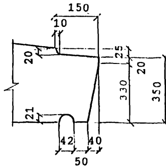
Конструкция концевой участка плиты балластного корыта 1:10
