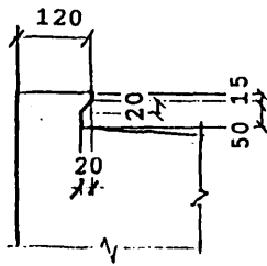
Деталь заделки изоляции 1:10
