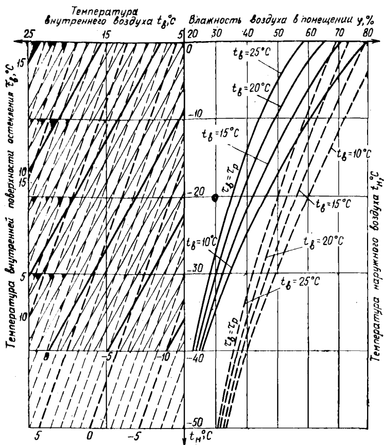
Рис 2. Номограмма для определения температур \tau_n , \tau_p и допустимых значений t_n , \phi при теплотехнических расчетах окон с применением стеклопакетов
