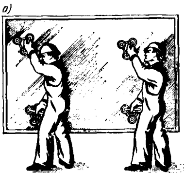
Рис. 10. Переноска стеклопакетов с помощью вакуум-присосок а — переноска; б — общий вид ручной вакуум-присоски
