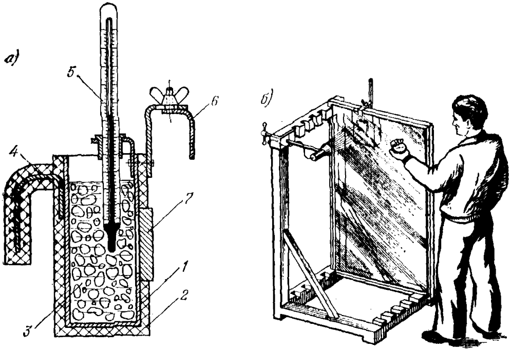
Рис. 14. Контроль точки росы в воздушной прослойке стеклопакета
