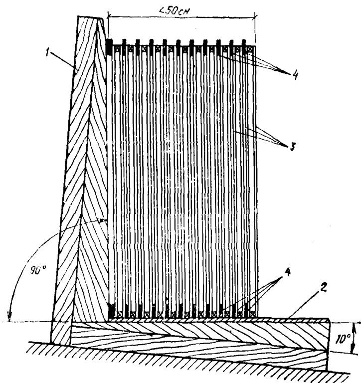
Рис. 9. Стеллаж для хранения стеклопакетов 1 — стеллаж; 2 — подкладка из войлока или резины; 3 — стеклопакеты; 4 — прокладки из войлока, картона или резины
