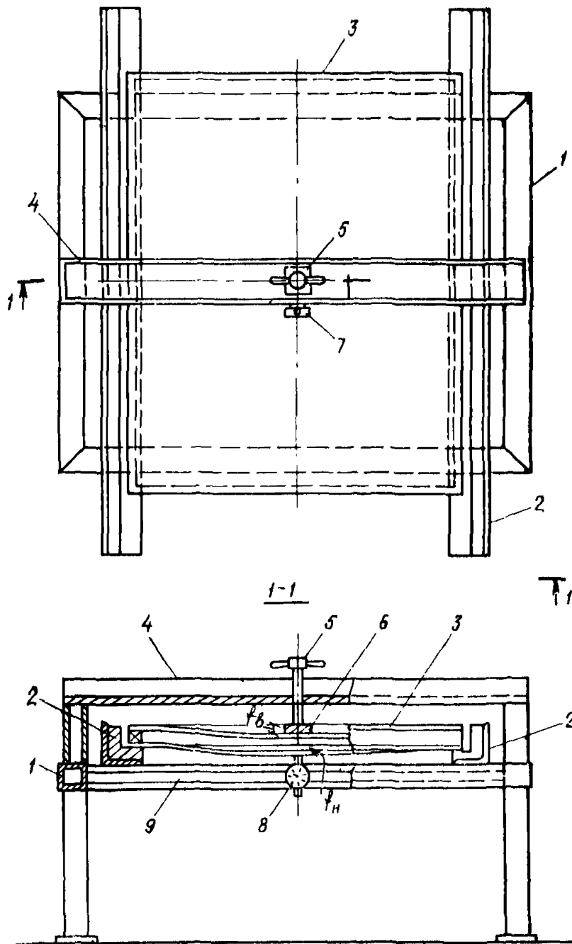
Рис. 13. Стенд для контроля герметичности стеклопакета 1 — рама; 2 — направляющая; 3 — стеклопакет; 4 — балка; 5 — винт; 6 — пластмассовая прокладка; 7 и 8 — индикаторы; 9 — рейка для крепления нижнего индикатора
