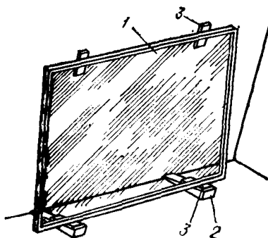
Рис. 11. Временное опирание стеклопакета при монтаже 1 — стеклопакет; 2 — деревянные подкладки; 3 — войлочные или резиновые прокладки
