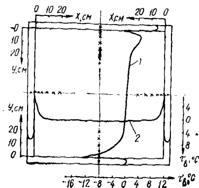
Рис. 16. Температурные поля на внутренней поверхности двухслойного стеклопакета и деревянного оконного переплета
