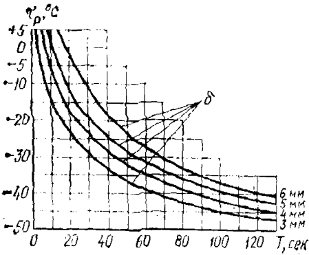
Рис. 15. График для определения точки росы t_p в зависимости от времени обнаружения T и толщины стекла \delta в стеклопакете
