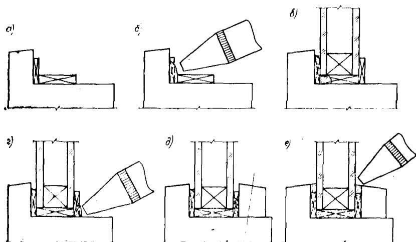
Рис. 12. Последовательность операций при установке стеклопакетов в переплете и герметизации зазоров нетвердеющей мастикой
