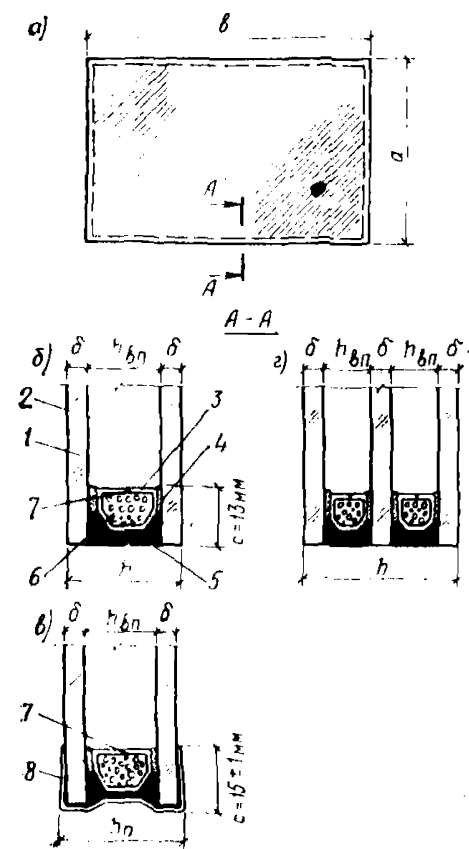
Рис. 1. Конструкция клееных стеклопакетов
