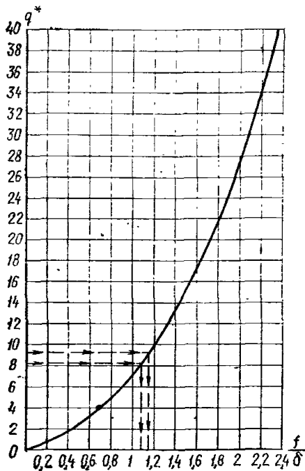
Рис. 5. График для определения прогиба наружного стекла f стеклопакета и отношения f/\delta от расчетной нагрузки
