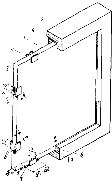
Рис. 6. Установка стеклопакета в переплете с использованием прокладок и нетвердеющей мастики
