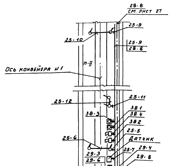
ПЛАН НА ОТМ. 7.200 М 1:100
