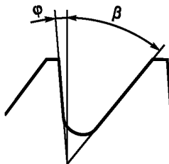
Рисунок 5 — Упорная резьба
