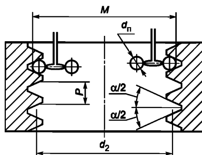
Рисунок 10 — Измерение среднего диаметра калибра-кольца
