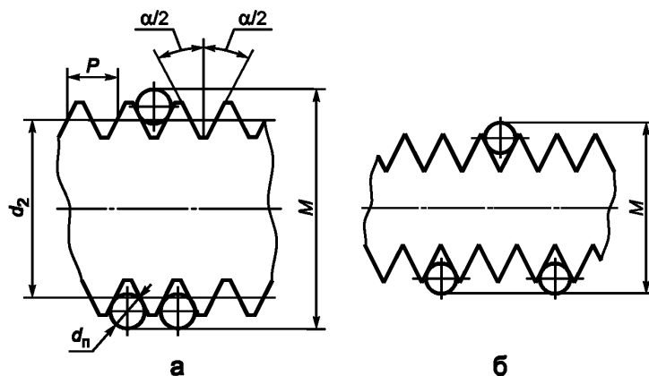
Рисунок 4 — Метод трех проволок
