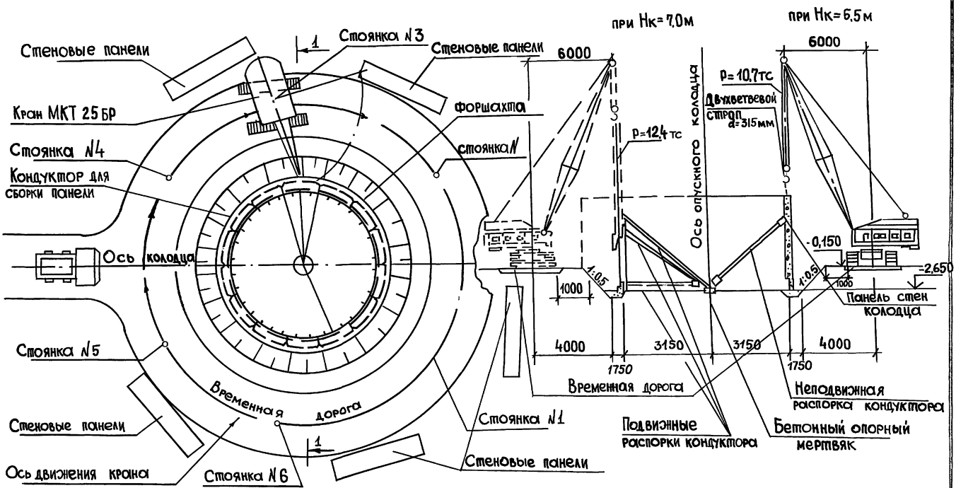
Разрез 1-1
