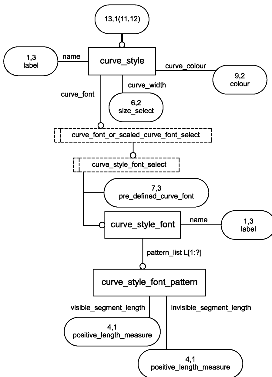
Рисунок С.13 — ПИК aic_mechanical_design_shaded_presentation в формате EXPRESS-G (диаграмма 13 из 16)
