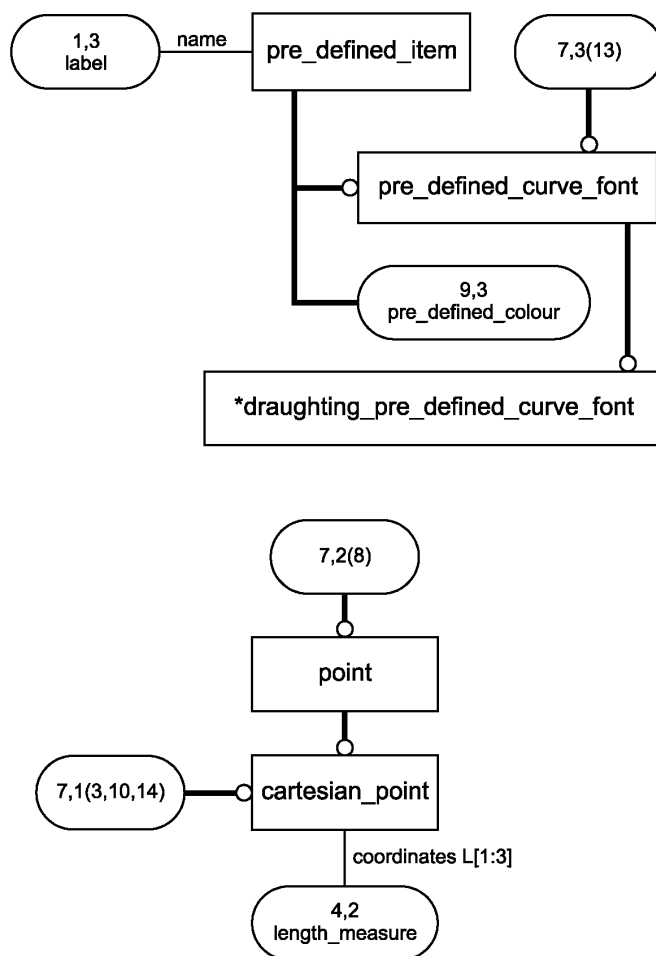
Рисунок С.7 — ПИК aic_mechanical_design_shaded_presentation в формате EXPRESS-G (диаграмма 7 из 16)
