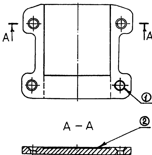
Рисунок 5.8. Планка фрикционная
