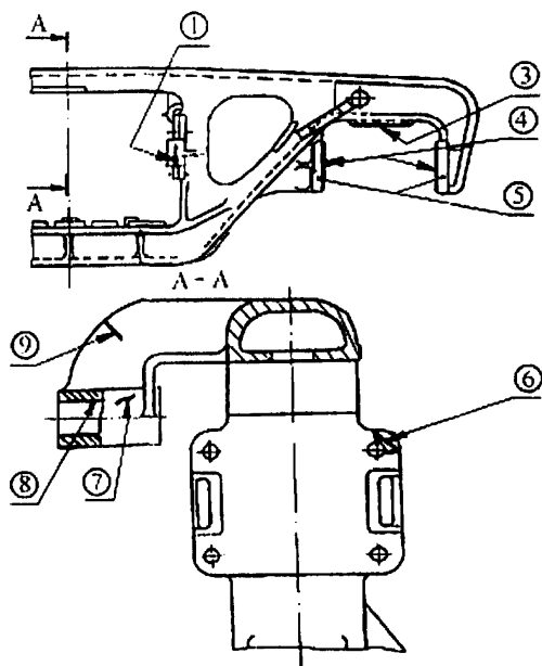
Рисунок 5.7. Рама боковая
