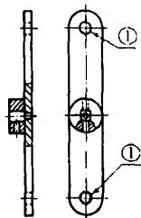
Рисунок 5.172. Рычаг
