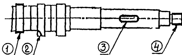
Рисунок 5.92. Вал распределительный
