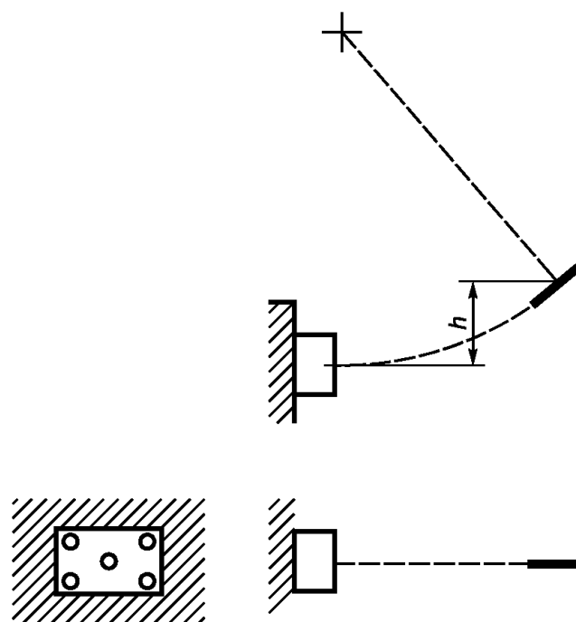
h — высота падения; \circ — точки нанесения ударов
