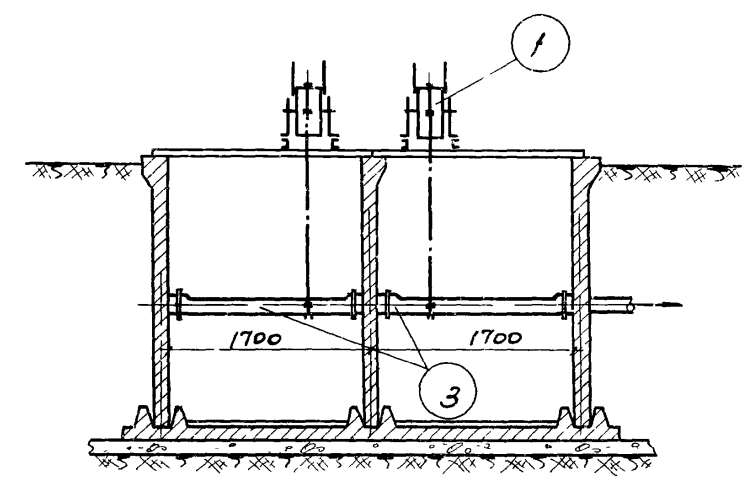
Б-Б М 150
