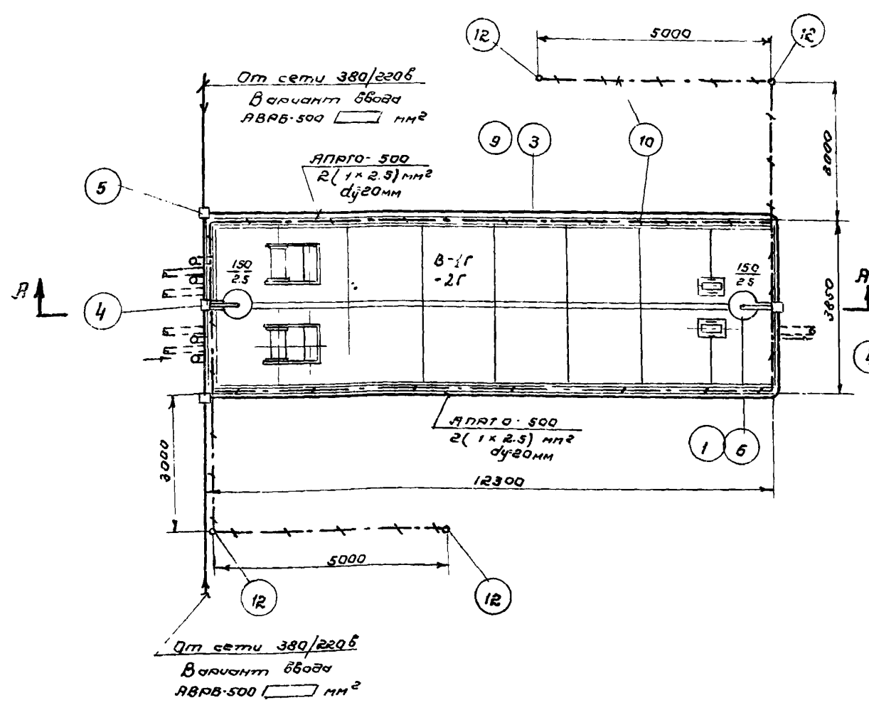
План М 1:100
