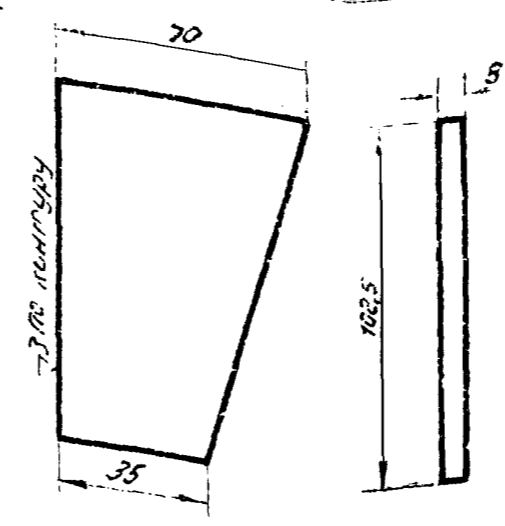
Деталь N 23
