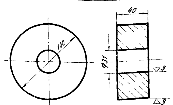
Деталь N 16
