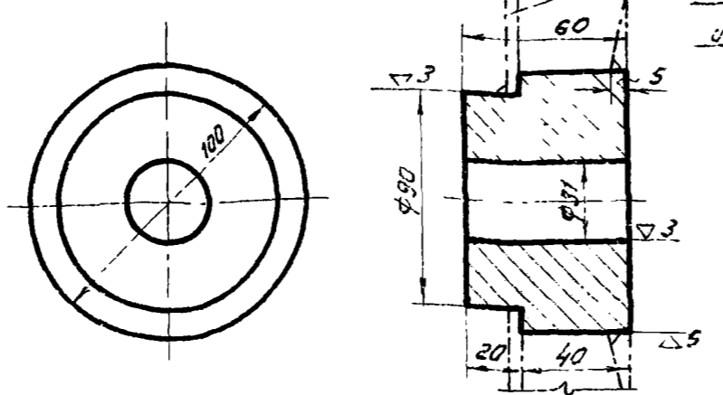
Деталь N 17
