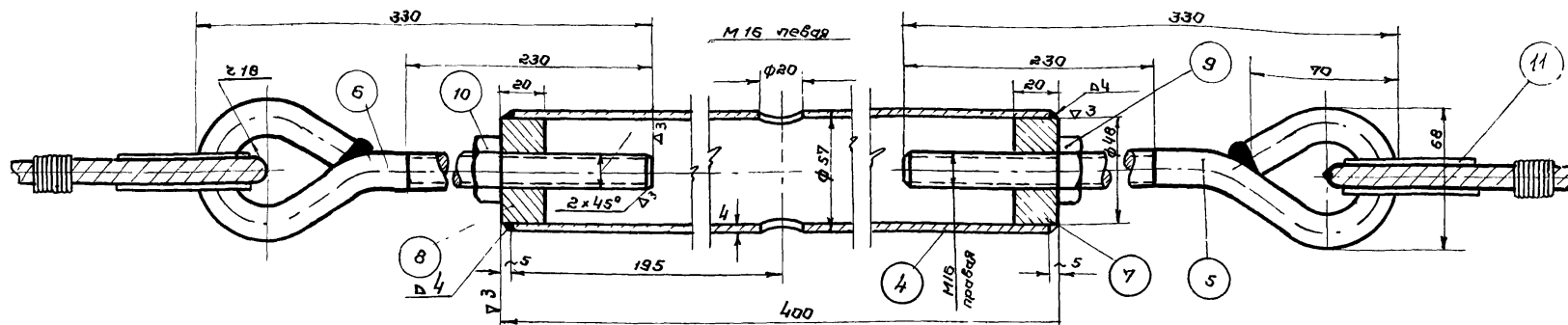
Стяжка (в сборе) М1:2
