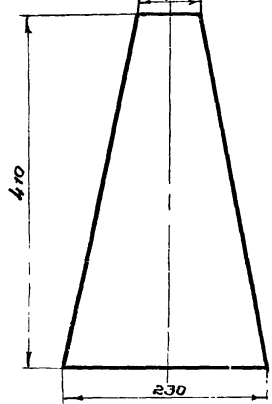
Деталь 1 М1:5
