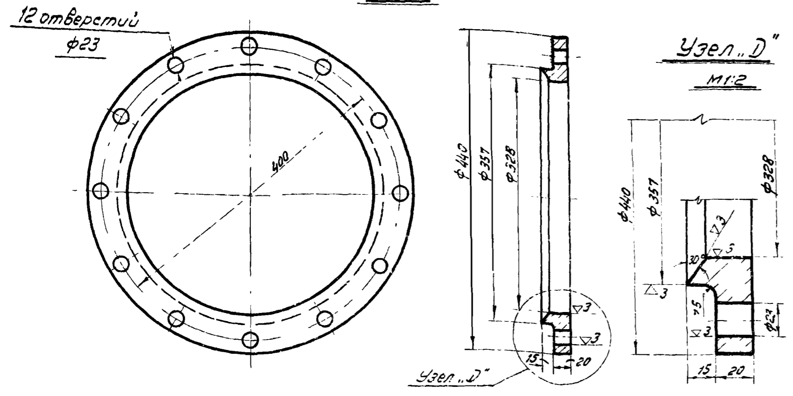
Деталь N 8
