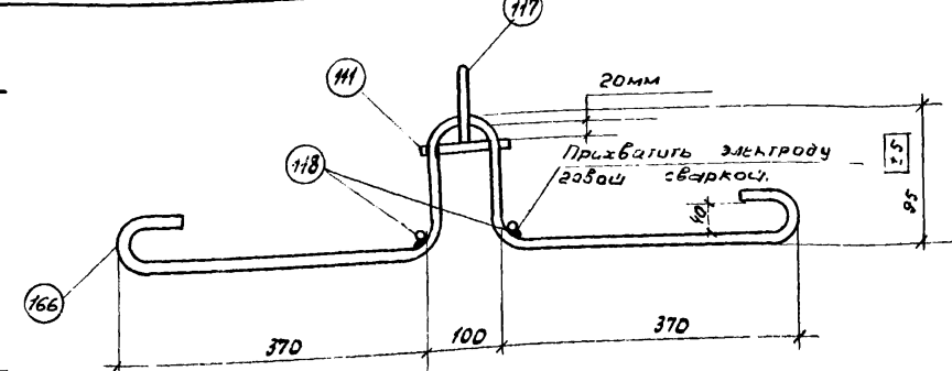
МОНТАЖНАЯ ПЕТЛЯ М-16
