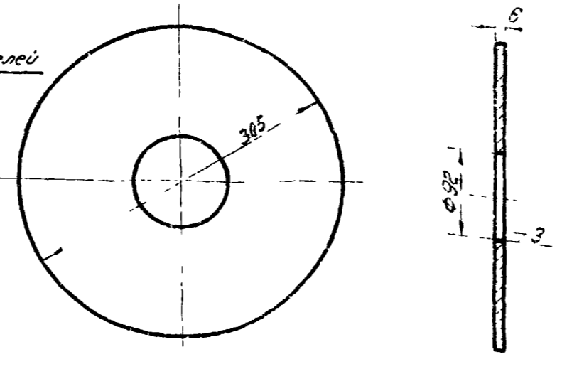
Деталь N 13
