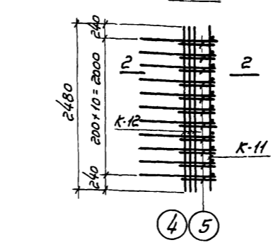
Пакет ПК-5
