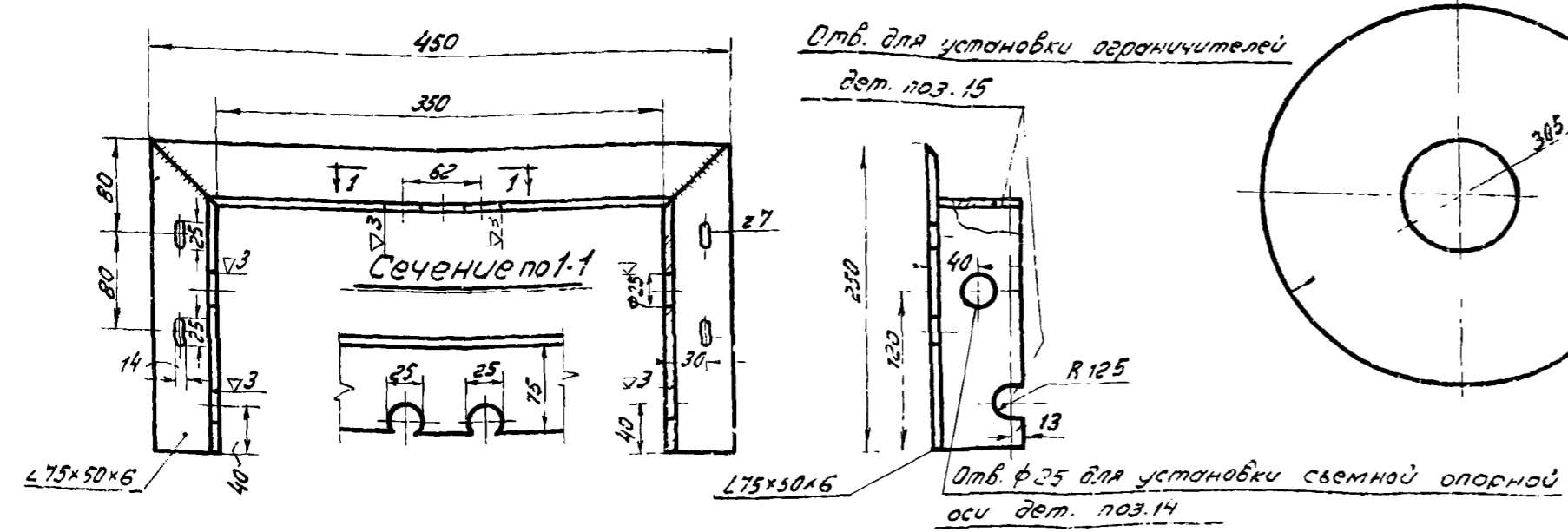
Деталь N 13
