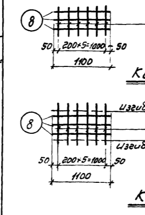
Пакет ПК-15
