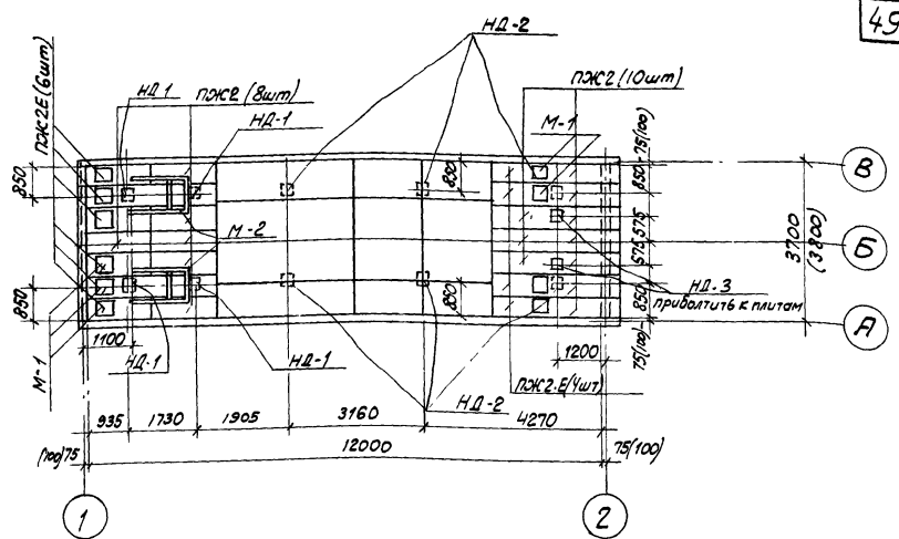
Расположение закладных в покрытии
