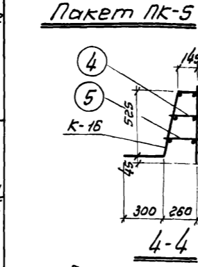
Пакет ПК-5
