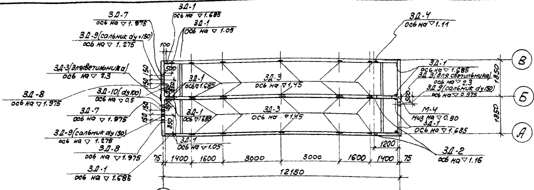
Расположение закладных в нефтеловушке с высотой панелей 2,4 м.
