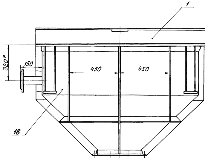
Вид Б лист 1 М 1:10
