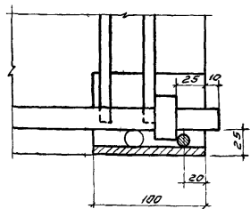
(Вариант с анкером, обжатая обойтка)
