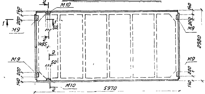
Марки плит с индексом "в"
