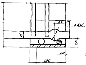
(Вариант с анкером, высаживная головка)
