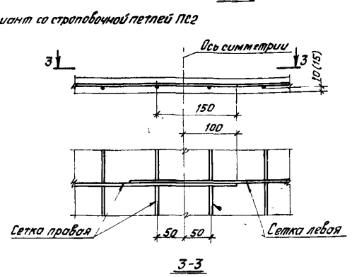
Деталь стыка сеток С10 - С40 (см. пункт 5 примечания)
