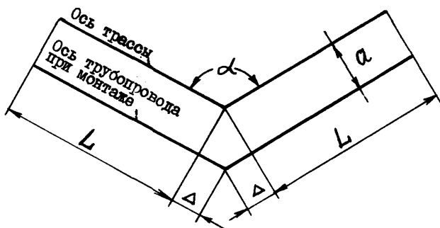
Рис.1. Прокладка трубопровода по традиционной схеме
