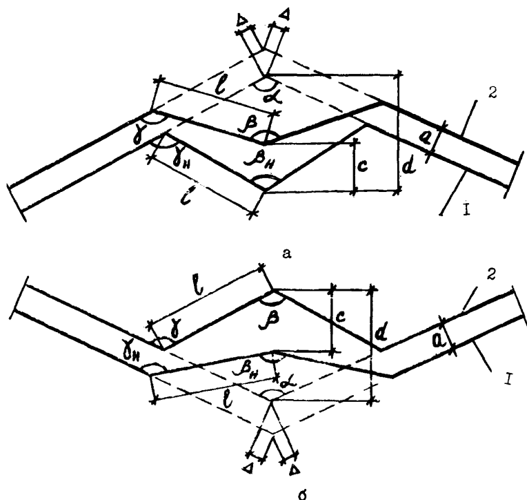
Рис.2. Схема прокладки трубопровода на криволинейном участке трассы с тремя углами:
