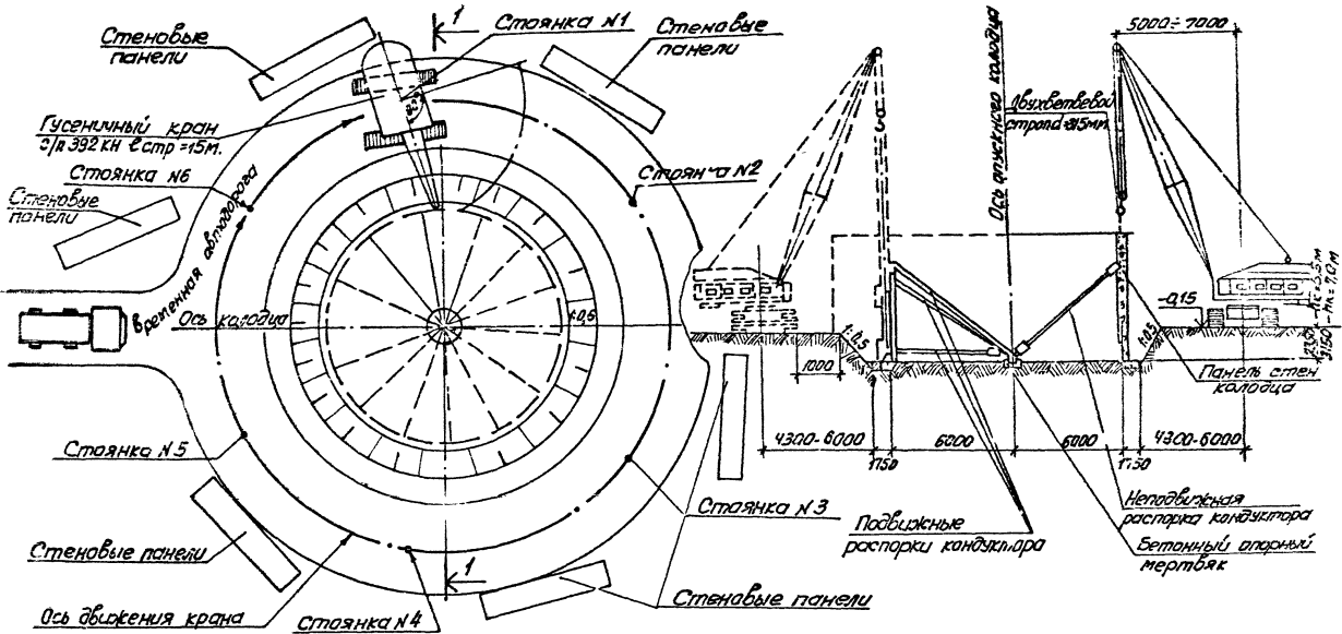
Схема монтажа стеновых панелей опускного колодца подземной части насосной станции.
