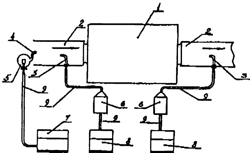
Схема контроля фильтра при работающей вентиляционной системе
