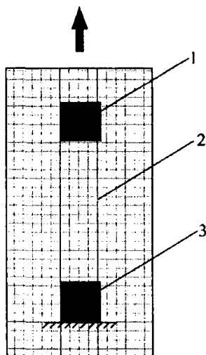
Рисунок 7.19 — Пример испытания на растяжение посредством захвата («Греб»-метод)
