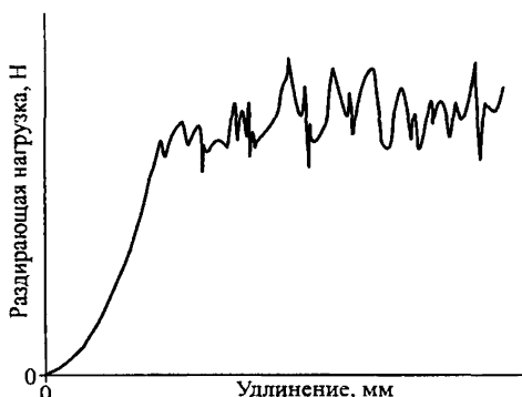
Рисунок 7.23 — Определение раздирающей нагрузки по диаграмме раздираания
