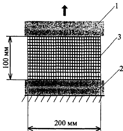
1,2 – зажимы; 3 – образец
