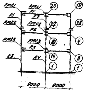
Поперечные (рабочая и связевая) рамы
