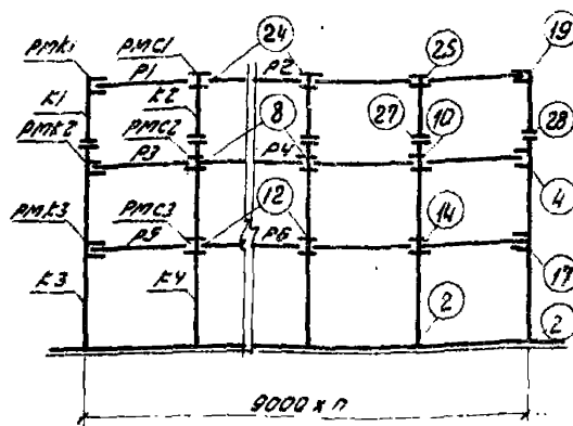
Поперечные (торцевая и у.а.ш.) рамы
