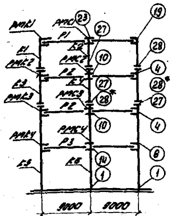
ПЕРЕКРЫТИЕ (РЯДОВЫЕ И СВЯЗЕВЫЕ) РАМЫ
