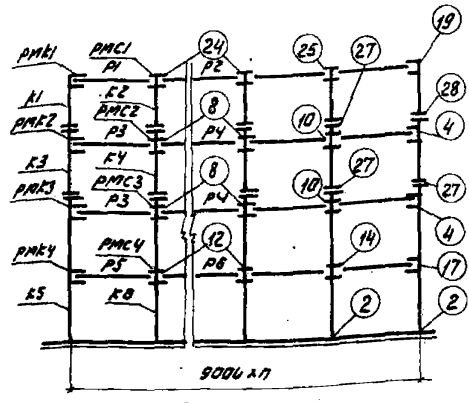
Поперечные (торцевая и У-образная) рамы
