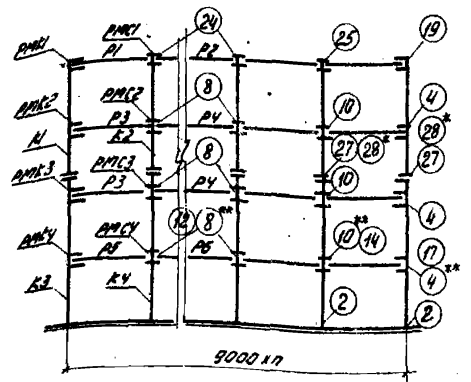
Поперечные (торцевая и угловая) рамы
