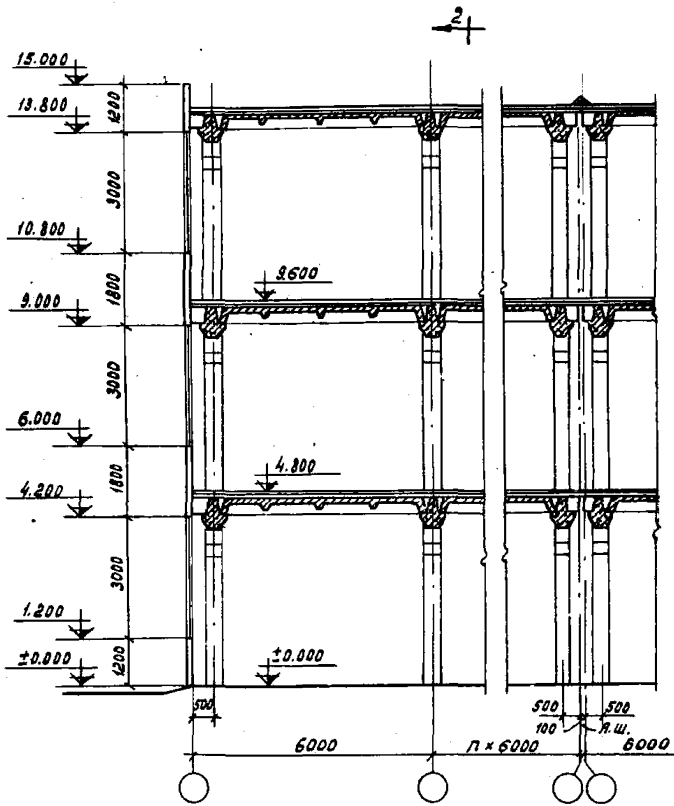
1-1 Продольный разрез (пример)
