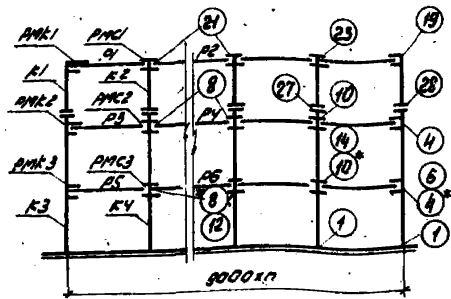
Поперечные (рабочая и связевая) рамы
