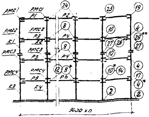
Поперечные (торцевая и у.ш.) рамы
