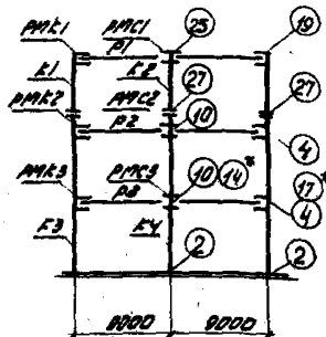
Поперечное (торцевая и ч.ч.ш) рамы
