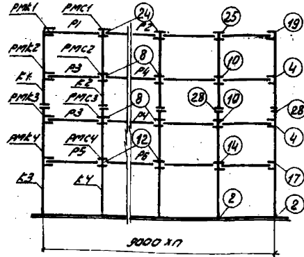
Поперечные (торцевая и з.ш.) рамы
