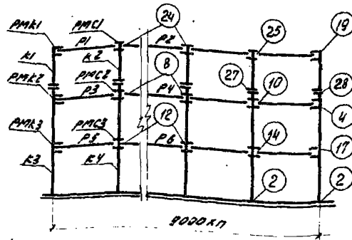
Поперечные (торцевая и у.ш.) рамы
