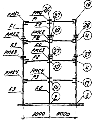
Поперечные (торцевая и з.н.ш.) рамы
