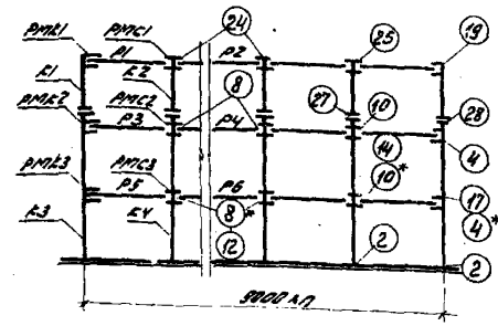
Поперечные (торцевая и у.ш.) рамы
