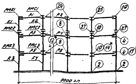
Перпендикулярные (торцевая и ч.л.ш.) рамы
