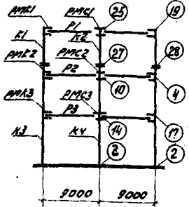
Поперечные (торцевая и чаш) рамы
