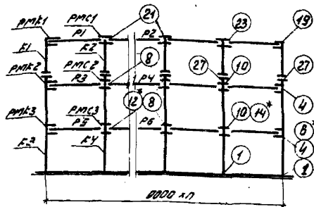
Перпендикулярные (рядовая и связевая) рамы
