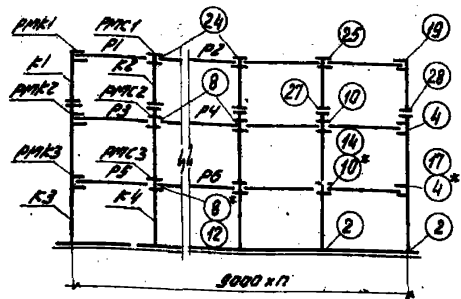
Поперечные (платформа и у.а.ш.) рамы
