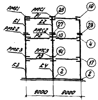
Поперечные (торцевая и у.в.ш.) рамы
