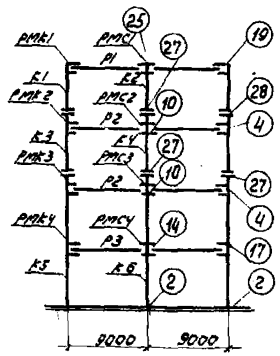
Поперечная (торцевая и уащ) рамы
