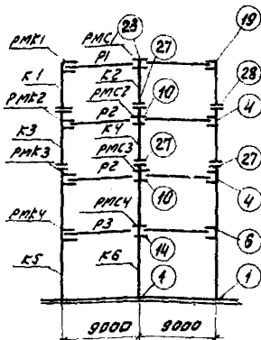
Поперечные (рядовая и связная) рамы
