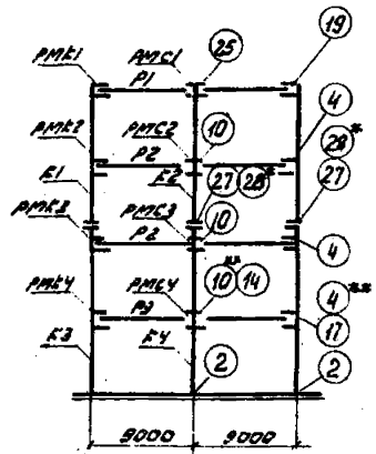
ПОПЕРЕЧНЫЕ (торцевая и У.Ш.) рамы
