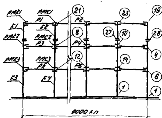
Поперечные (рядовая и связевая) рамы
