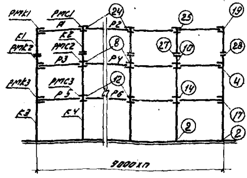
Поперечные (торцевая и ч.л.ш.) рамы
