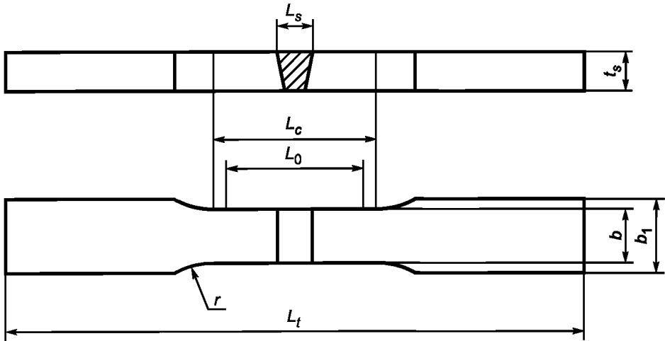
а) образцы для испытаний сварных соединений пластин
