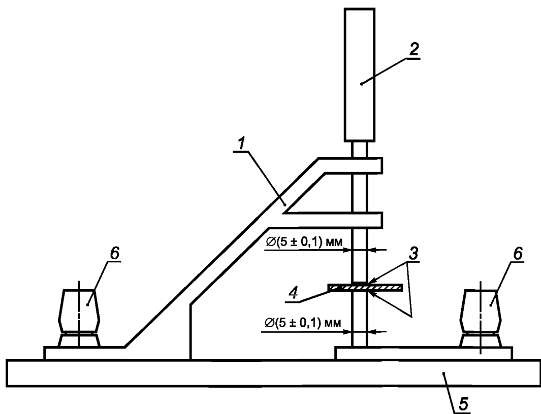
1 — металлическая рама, удерживающая штырь в вертикальном положении (штырь свободно движется в вертикальном направлении); 2 — металлический штырь массой 100 г; 3 — края штыря закруглены радиусом 0,5 мм; 4 — испытуемый образец; 5 — изоляционное основание; 6 — клеммы для подачи испытательного напряжения
