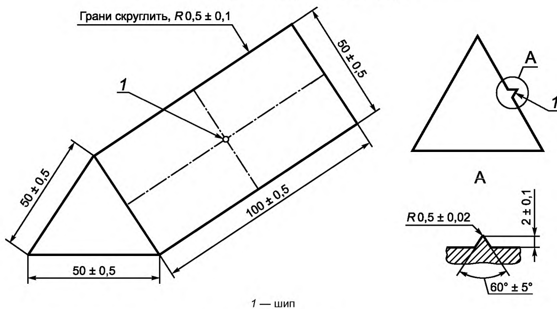
Рисунок 14 — Оправка
