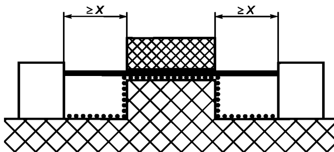
Рисунок E.5 — Несплошной стык с узкими канавками
