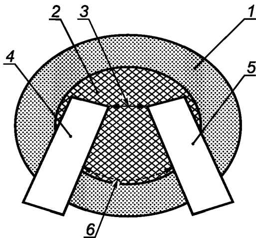
1 — изоляционная оболочка; 2 — изоляционный компаунд; 3 — расстояние через изоляцию; 4 — проводящая часть 1; 5 — проводящая часть 2; 6 — потенциальный зазор и путь утечки вдоль стыка
