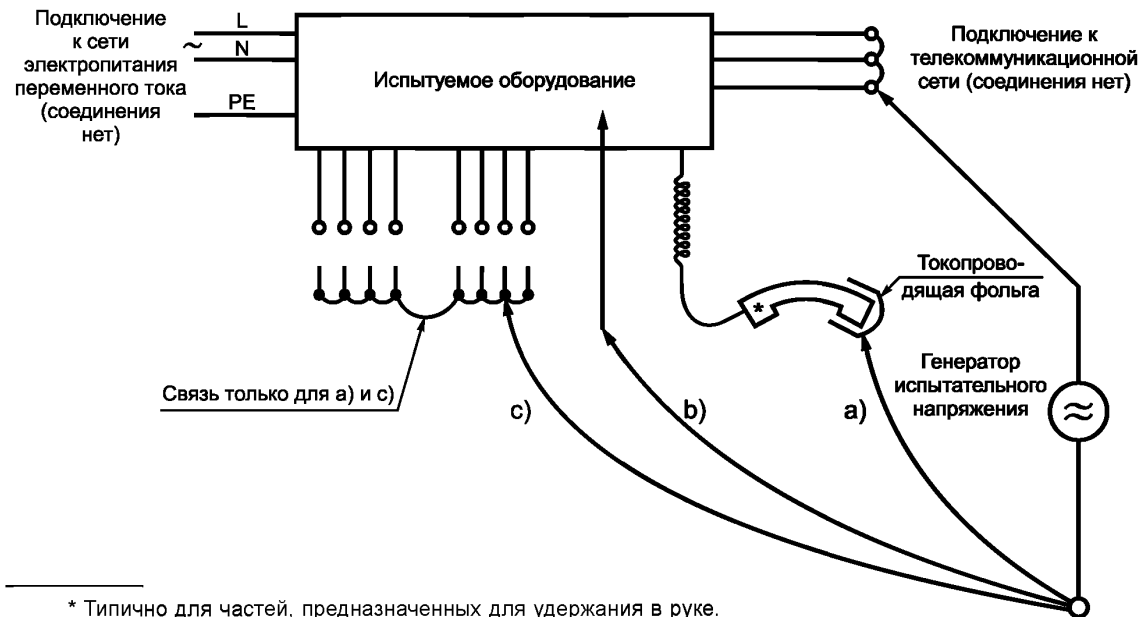
Рисунок 6В — Точки приложения испытательного напряжения
