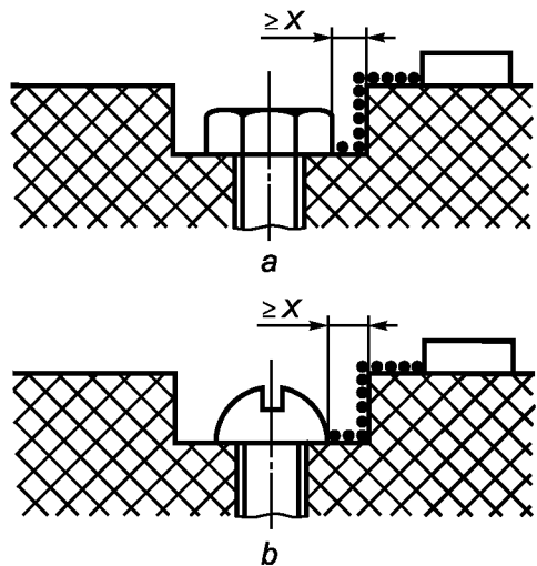
Рисунок F.8 — Малое углубление
