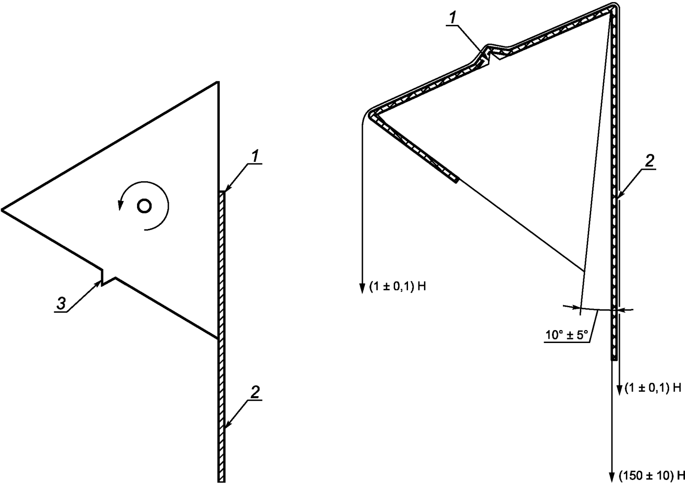
1 — крепежный элемент; 2 — изоляционный материал; 3 — шип
