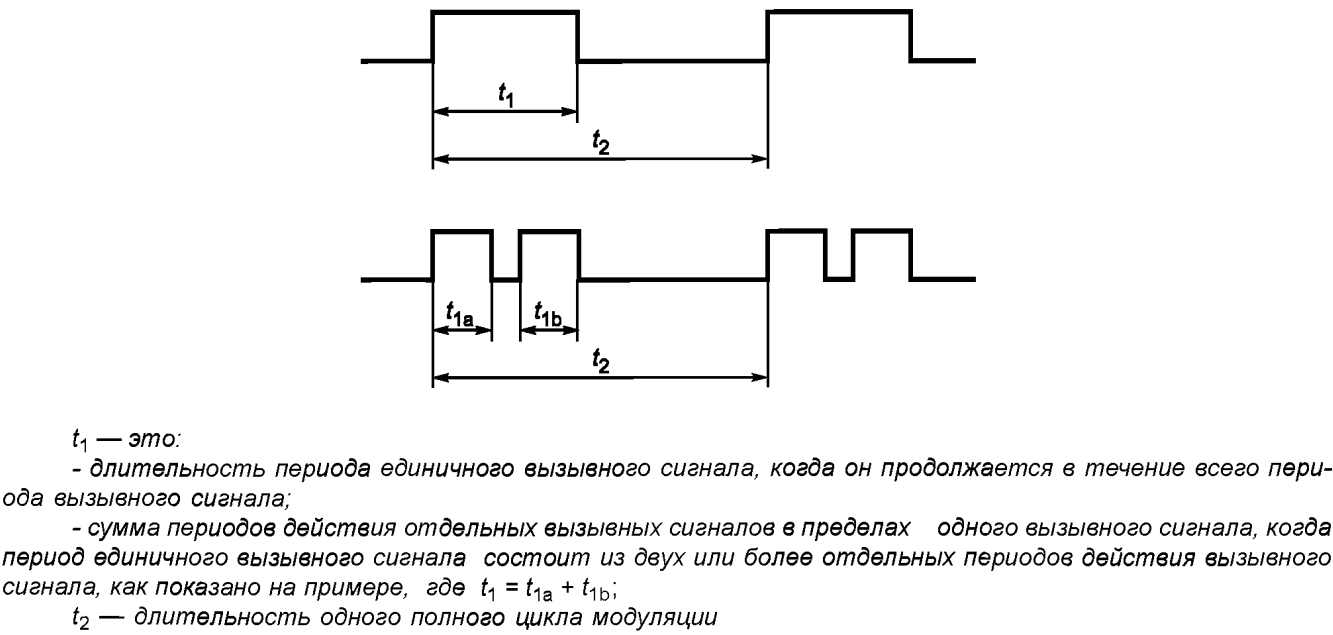
Рисунок М.1 — Определение длительности периода вызывного сигнала и цикла модуляции
