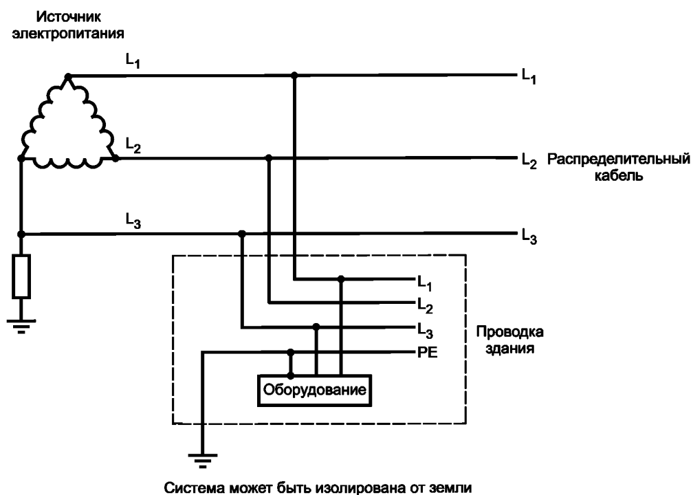
Рисунок V.8 — Пример IT-системы электропитания с тремя фазами
