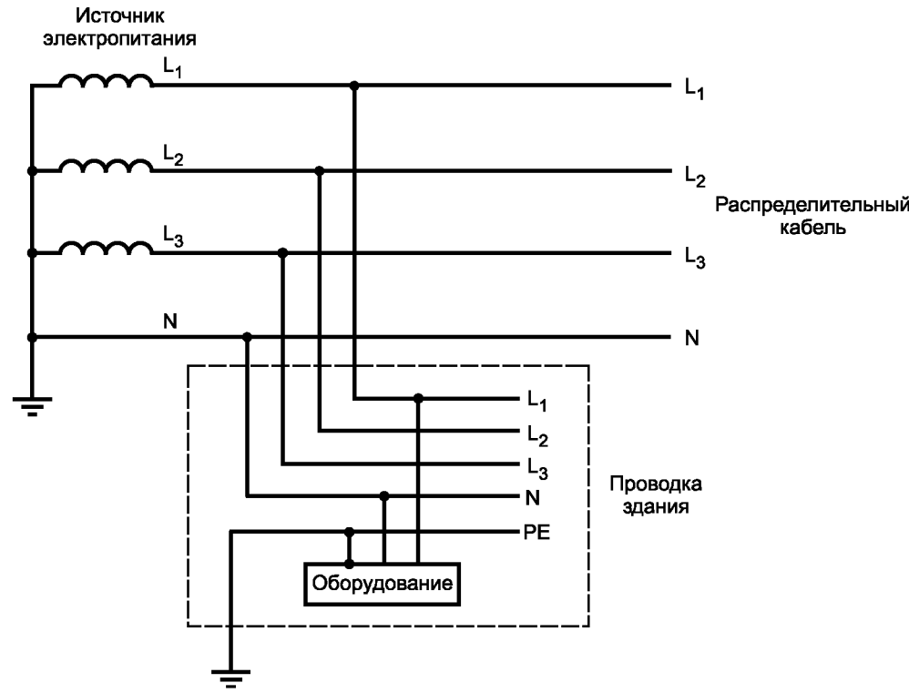
Рисунок V.5 — Пример TT-системы электропитания с тремя фазами и нейтралью
