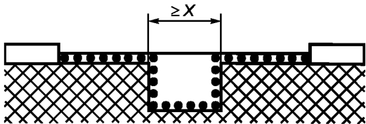
Рисунок F.1 — Узкая канавка
