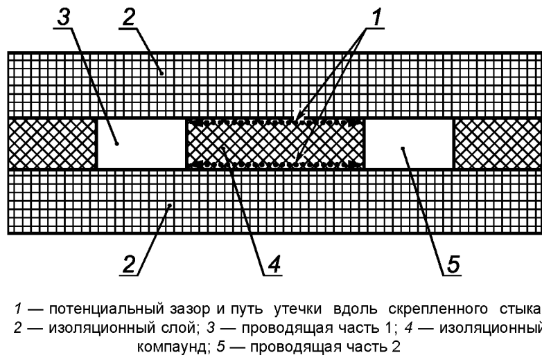
Рисунок F.15 — Тонколистовой изоляционный материал
