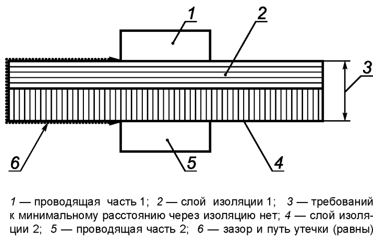
Рисунок F.14 — Сплошной изоляционный материал
