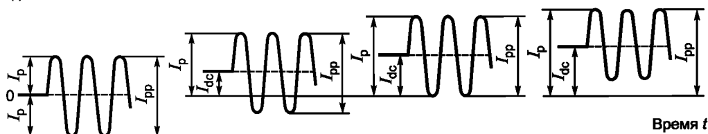
Рисунок М.3 — Двойная амплитуда тока и пиковое значение тока относительно земли
