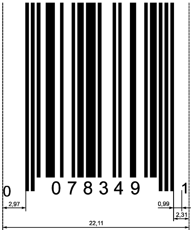
Рисунок E.5 — Символ UPC-E
