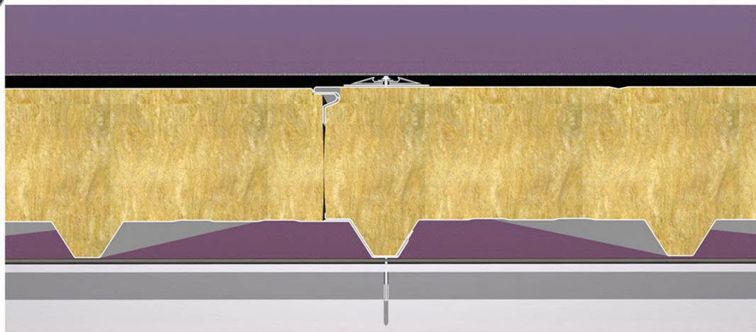
Крепление мембраны с помощью системы KLEMMFIX
