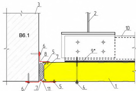
СТЫК С СУЩЕСТВУЮЩЕЙ СТЕНОЙ В6.1,6.2
