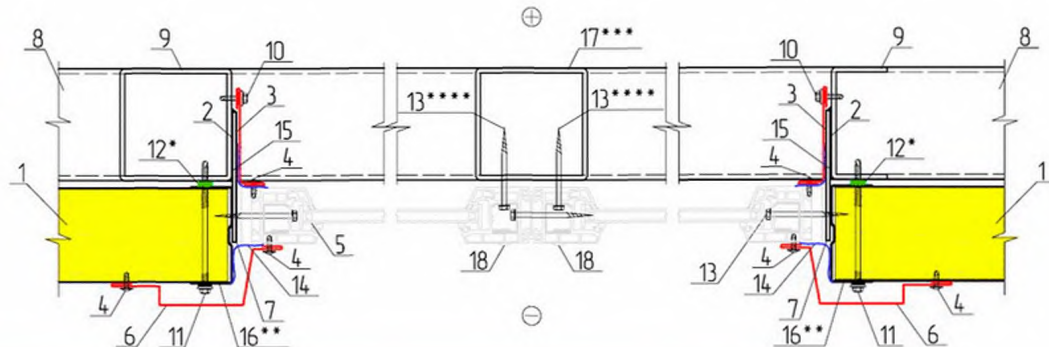
КРЕПЛЕНИЕ ОКОННОГО БЛОКА В1.4
