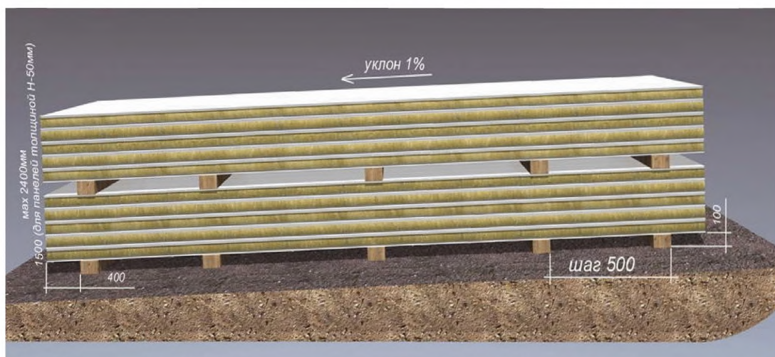
Рисунок 11 – Схема складирования пакетов панелей
