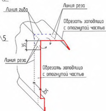
Схема подреза
