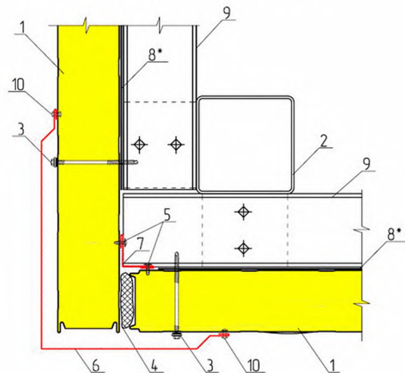
УГОЛ ЗДАНИЯ НАРУЖНЫЙ ВЗ.1
