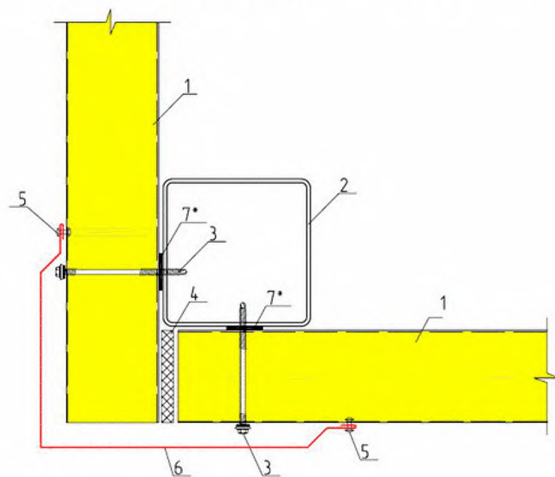
УГОЛ ЗДАНИЯ НАРУЖНЫЙ ГЗ.1
