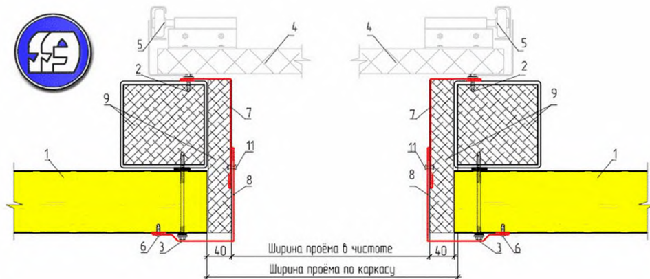
УЗЕЛ КРЕПЛЕНИЯ ПОДЪЕМНЫХ ВОРОТ ГОРИЗОНТАЛЬНЫЙ РАЗРЕЗ Г.В8.2
