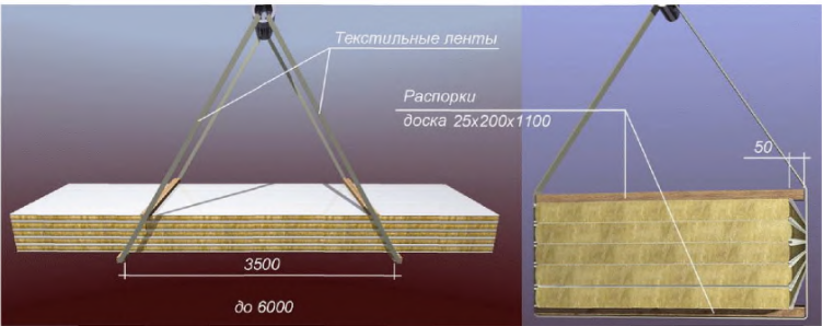
Рисунок 8 – Схема строповки пакетов панелей длиной не более 6000 мм
