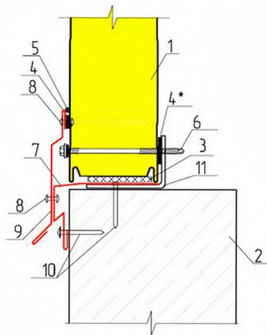
ЦОКОЛЬНЫЙ УЗЕЛ Г2.2
