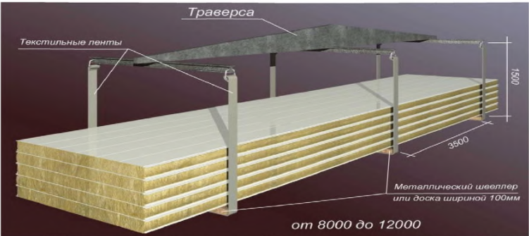
Рисунок 10 – Схема строповки пакетов панелей длиной более 8000 мм
