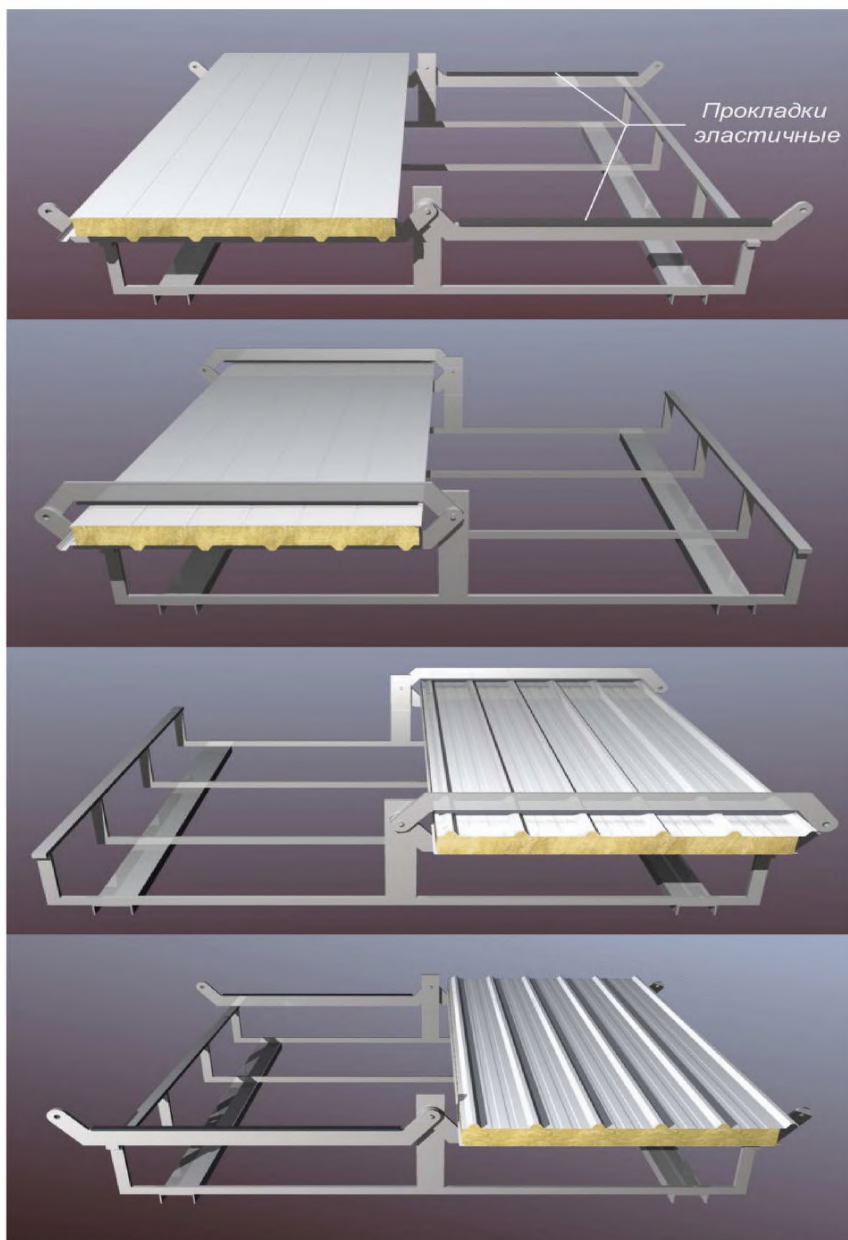
Рисунок 12д – Последовательность переворачивания кровельной панели на специальном столе для переворачивания.
