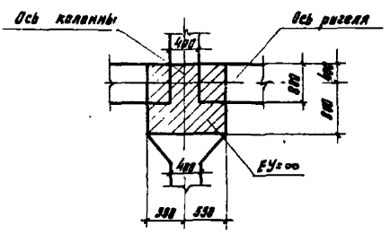
Участки повышенной жесткости в местах сопряжения ригелей со средними колоннами.
