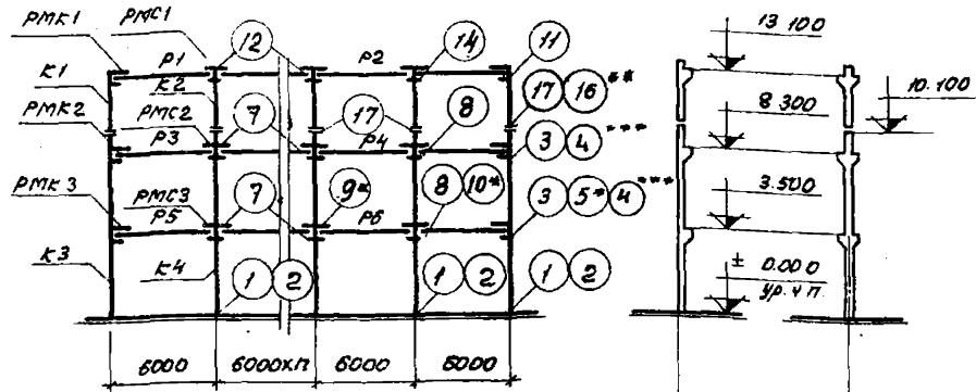
Поперечные (рядовая, связевая, торцевая и у а.ш.) рамы
