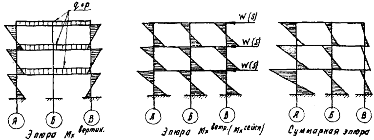
Рис. 5. Схематические эпюры моментов в колоннах поперечных рам.
