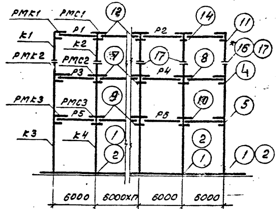
Поперечные (рядовая, связевая торцевая и у.ш.) рамы
