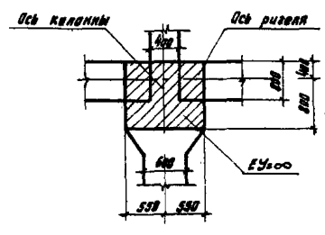
Участки повышенной жесткости в местах сопряжения ригелей со средними колоннами.
