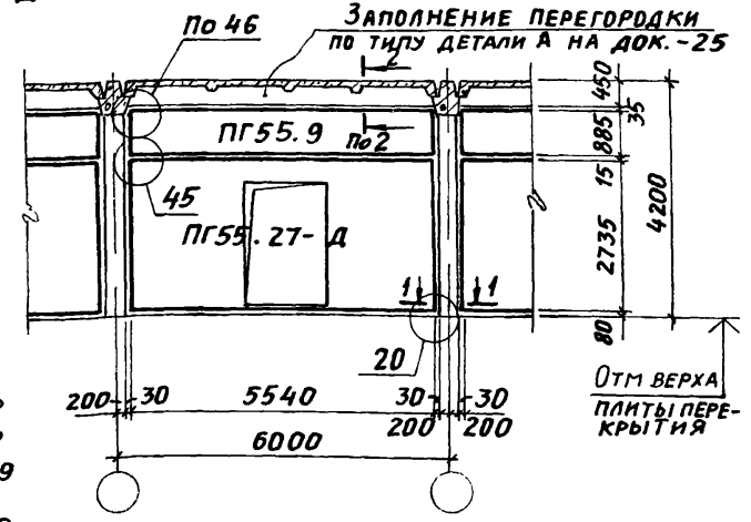
ПРОДОЛЬНАЯ ПЕРЕГОРОДКА В СТВОРЕ КОЛОНН КАРКАСА ЗДАНИЯ ДЛЯ СРЕДНЕГО И ВЕРХНЕГО ЭТАЖА
