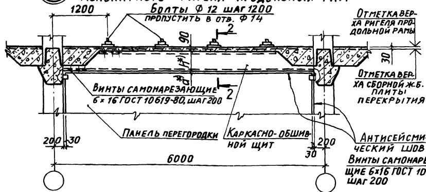
Б ВАРИАНТ ЗАПОЛНЕНИЯ ЗАЗОРА НАД ПЕРЕГОРОДКОЙ В ПРЕДЕЛАХ МОНОЛИТНОГО РИГЕЛЯ ПРОДОЛЬНОЙ РАМЫ
