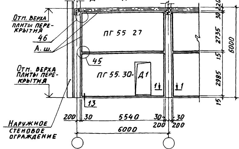
ПРОДОЛЬНАЯ ПЕРЕГОРДКА НЕ В СТВОРЕ КОЛОНН КАРКАСА ЗДАНИЯ ДЛЯ СРЕДНЕГО И ВЕРХНЕГО ЭТАЖА
