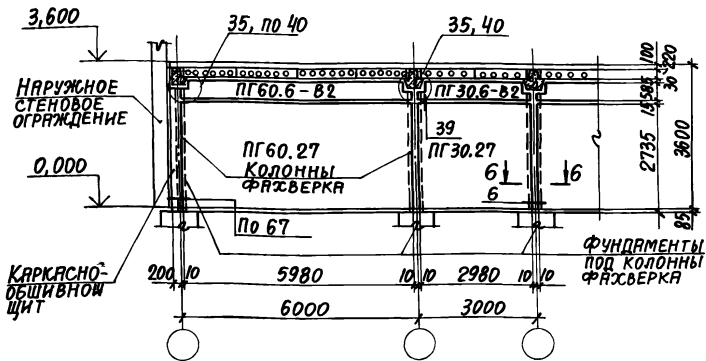
Сечение 1-1 см. л.1, сечение 6-6 см. л.5 док.-12
