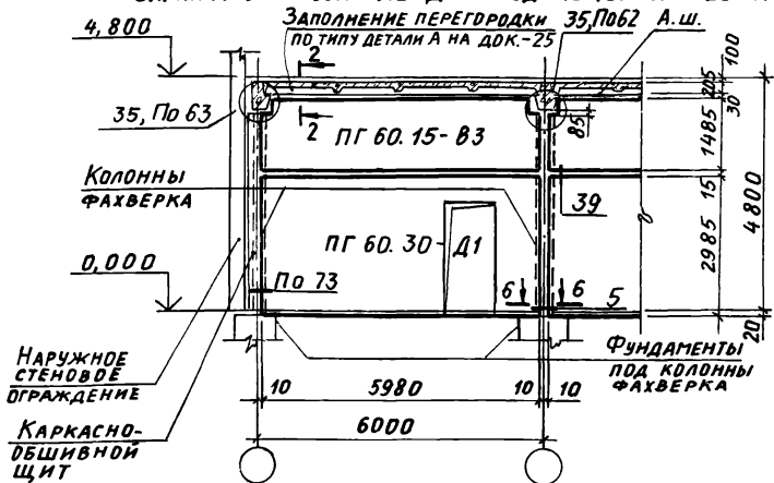
ПРОДОЛЬНАЯ ПЕРЕГОРДКА НЕ В СТОРЕ КОЛОНН ВАРИАНТ УСТАНОВКИ МЕЖДУ ПРОДОЛЬНЫМИ РЕБРАМИ
