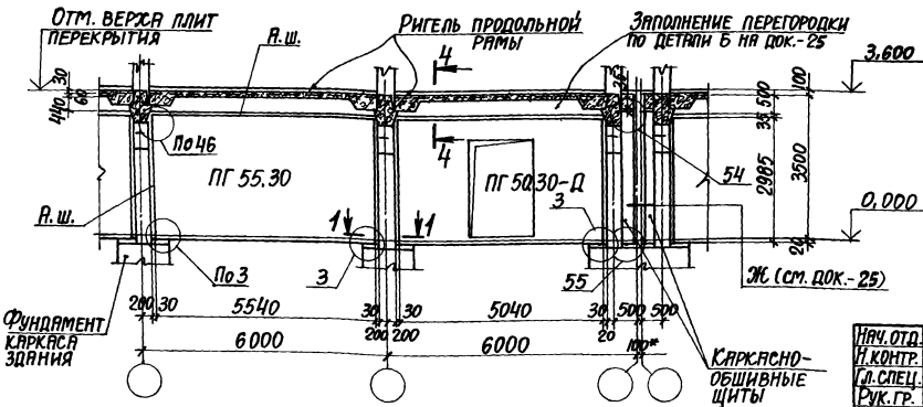
ПРОДОЛЬНАЯ ПЕРЕГОРОДКА В СТВОРЕ КОЛОНН КАРКАСА ЗДАНИЯ ДЛЯ ПЕРВОГО ЭТАЖА
