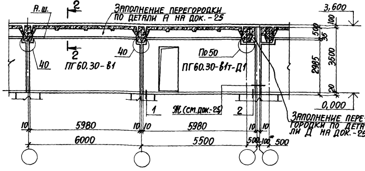
ПРОДОЛЬНАЯ ПЕРЕГОРОДКА В СТВОРЕ КОЛОНН КАРКАСА ЗДАНИЯ ДЛЯ ПЕРВОГО ЭТАЖА
