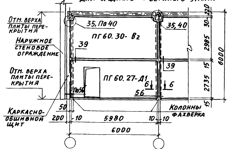
ПРОДОЛЬНАЯ ПЕРЕГОРДКА НЕ В СТВОРЕ КОЛОНН КАРКАСА ЗДАНИЯ ДЛЯ СРЕДНЕГО И ВЕРХНЕГО ЭТАЖА
