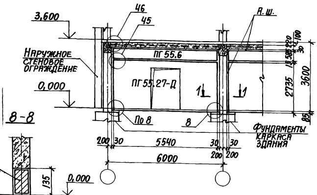
ПРОДОЛЬНАЯ ПЕРЕГОРОДКА НЕ В СТОРЕ КОЛОНН КАРКАСА ЗДАНИЯ ДЛЯ ПЕРВОГО ЭТАЖА
