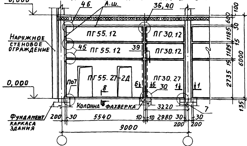
ПОПЕРЕЧНАЯ ПЕРЕГОРОДКА НЕ В СТВЕРЕ КОЛОНН КАРКАСА ЗДАНИЯ ДЛЯ ПЕРВОГО ЭТАЖА. ПРОЛЕТ L = 9 м
