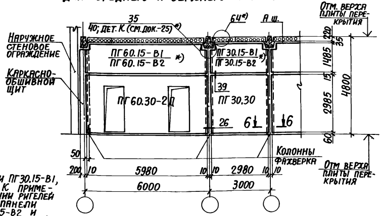
ПОПЕРЕЧНАЯ ПЕРЕГОРОДКА НЕ В СТВОРЕ КОЛОНН КАРКАСА ЗДАНИЯ ПРИ НАЛИЧИИ ПРОДОЛЬНЫХ РИГЕЛЕЙ ДЛЯ СРЕДНЕГО И ВЕРХНЕГО ЭТАЖА
