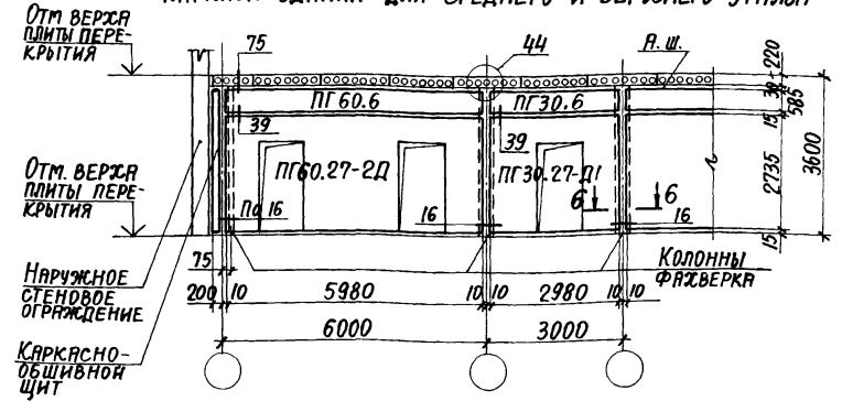
СЕЧЕНИЕ 1-1 СМ. Л. 1, СЕЧЕНИЕ 6-6 СМ. Л. 5 ДОК. - 12
