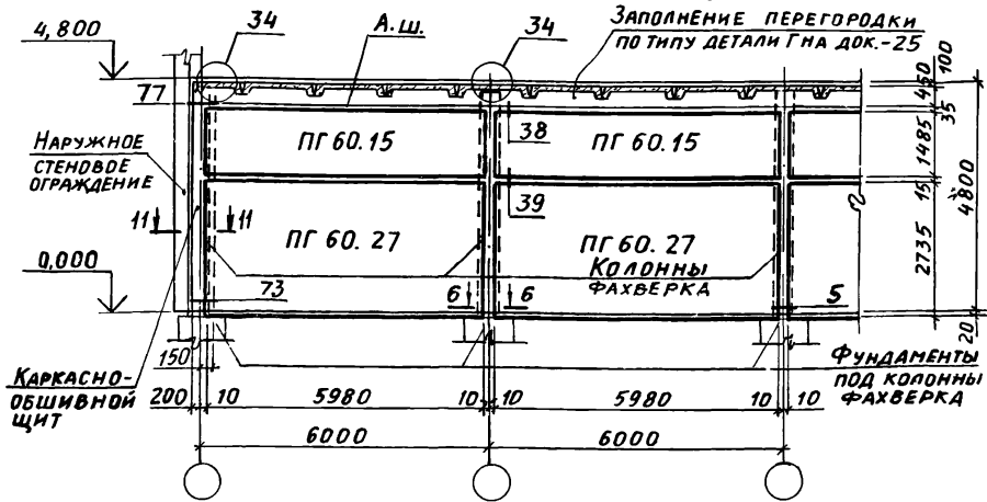
ПРОДОЛЬНАЯ ПЕРЕГОРДКА НЕ В СТОРЕ КОЛОНН ВАРИАНТ УСТАНОВКИ МЕЖДУ ПРОДОЛЬНЫМИ РЕБРАМИ
