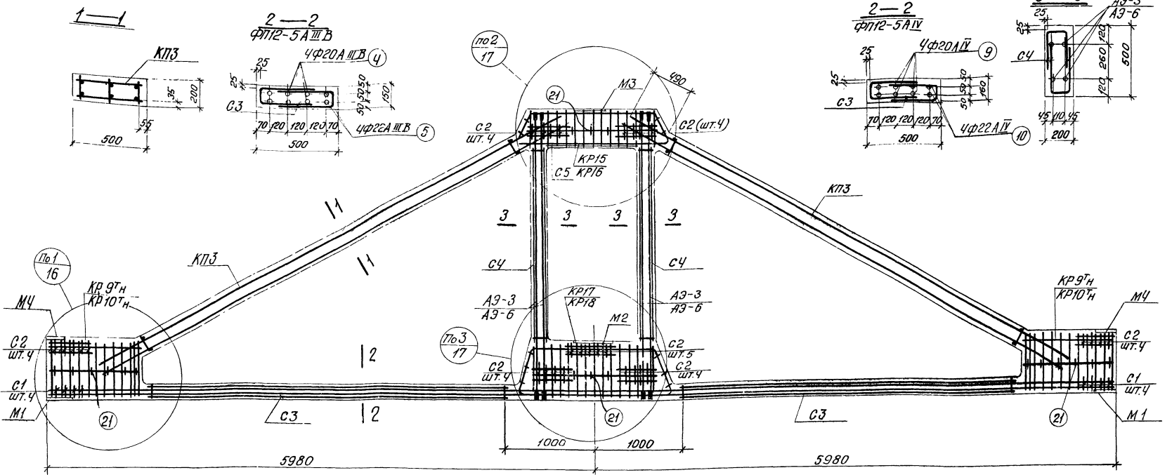
Контролируемое усилие натяжения напрягаемой арматуры
