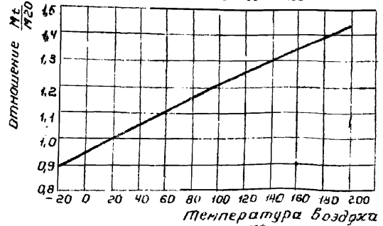
Рис.4. Зависимость отношения \frac{E_{ж}}{L \cdot 20} от температуры воздуха
