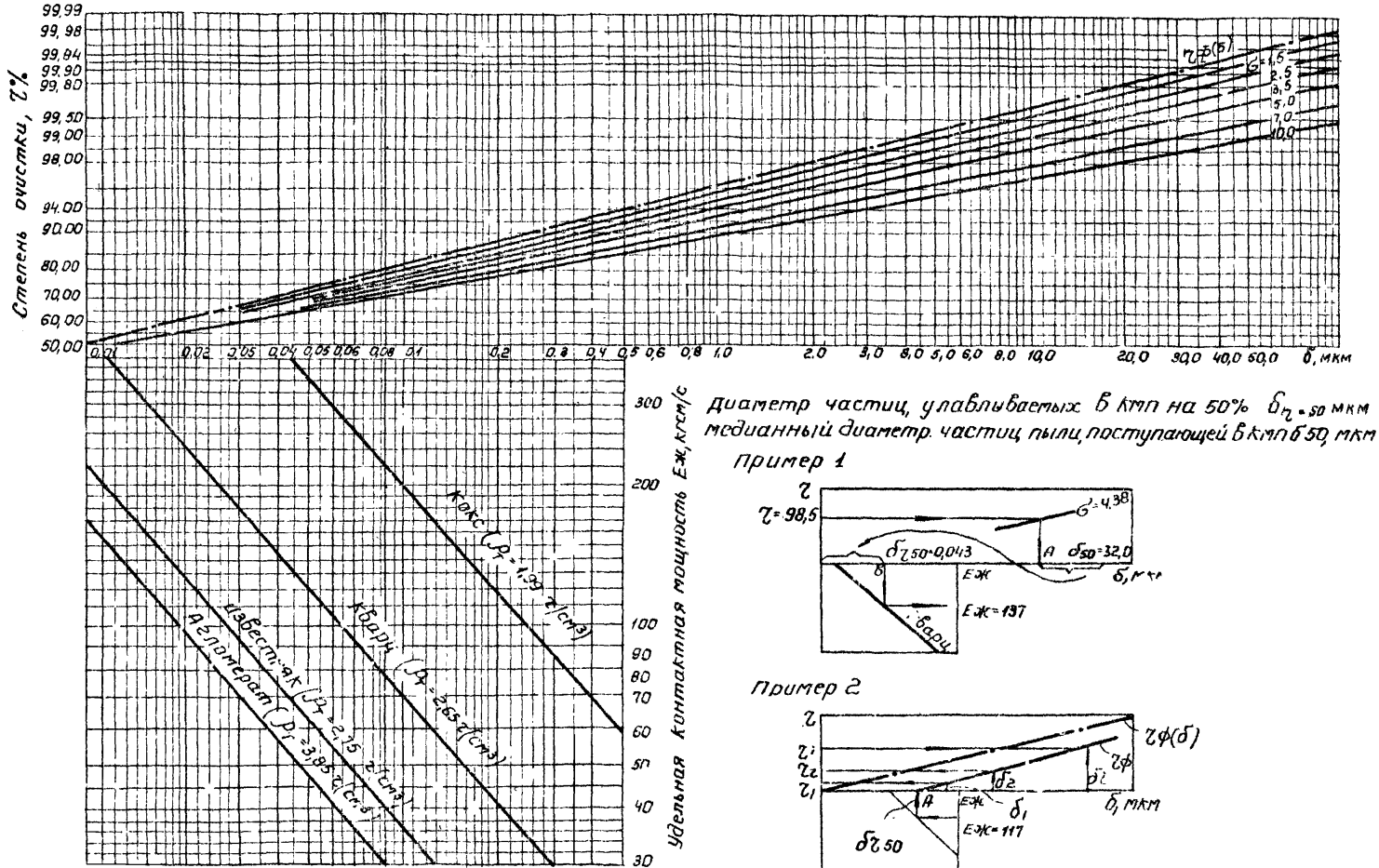
рис.2. Номаграмма зависимости удельной-контактной мощности ЕЖ от степени очистки, характеристик и типов пыли.
