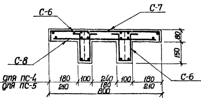
5-5 (для ПС-5)
