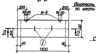
ПС-2
