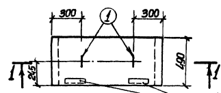
ПС-1, ПС-1А
