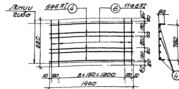
C-4
