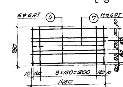
C-5
