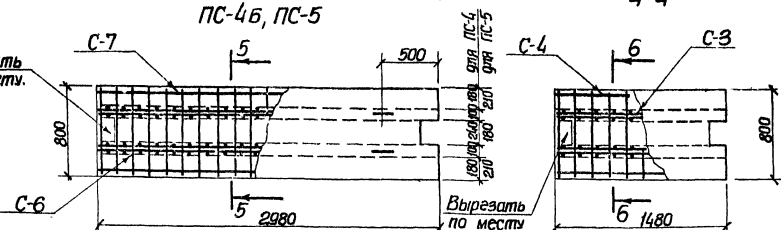
Армирование ПС-4, ПС-5
