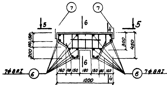
Армирование БС-1
