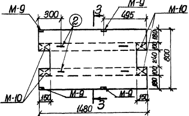
ПС-3
