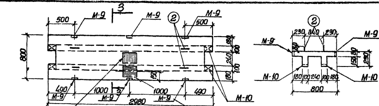
ПС-4, ПС-4А, ПС-4В
