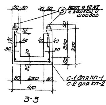
КП-1
