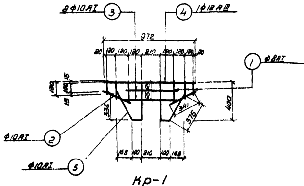
Кр-1
