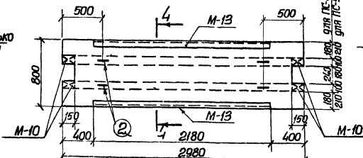
ПС-4Б, ПС-5
