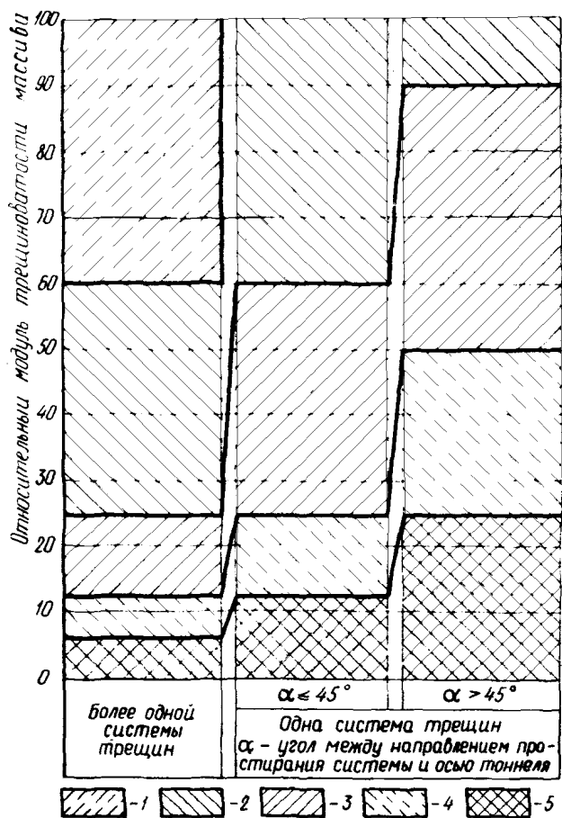
Рис.4. Диаграмма трещиноватости пород:
