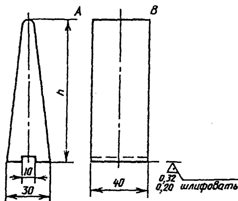
Опорные призмы
