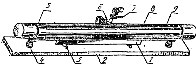
1—поверяемая линейка; 2—поверочная плита; 3—опоры; 4—домкраты; 5—оптическая линейка; 6—измерительная каретка; 7—микрометрический винт; 8—шанс оптической линейки; 9—шкала оптической линейки
